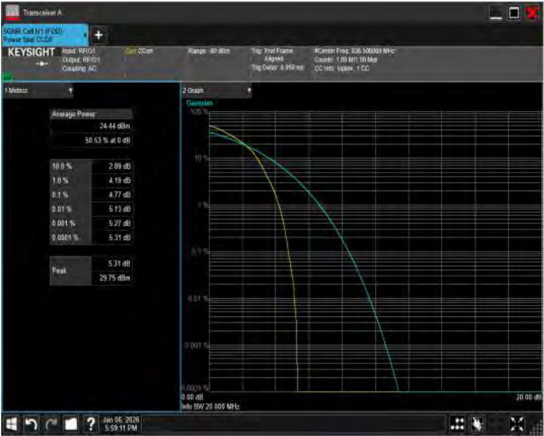
n26(824-849) SCS=15kHz DFT 64QAM BW=15MHz Channel=167300 RB=75@0
