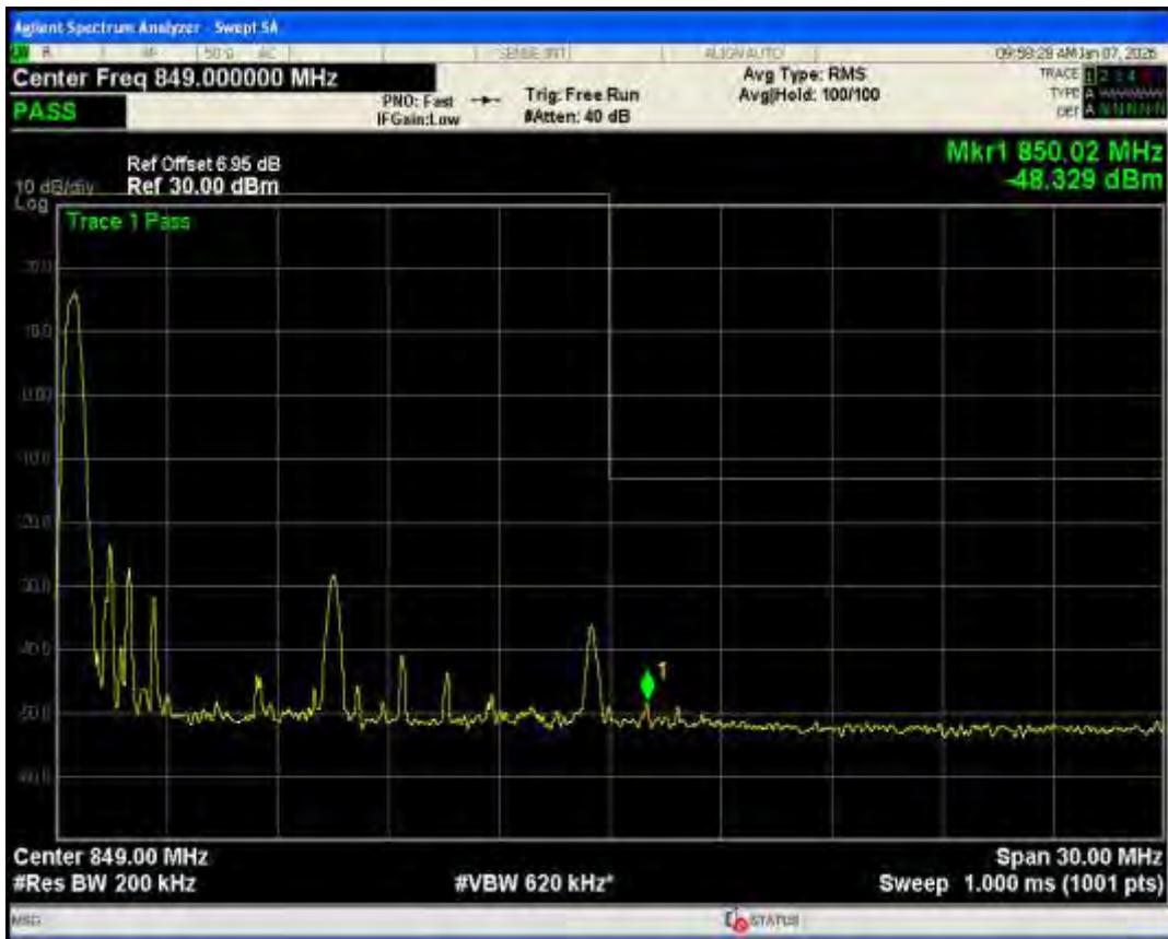
n26(824-849) SCS=15kHz CP QPSK BW=15MHz Channel=168300 RB=1@78
