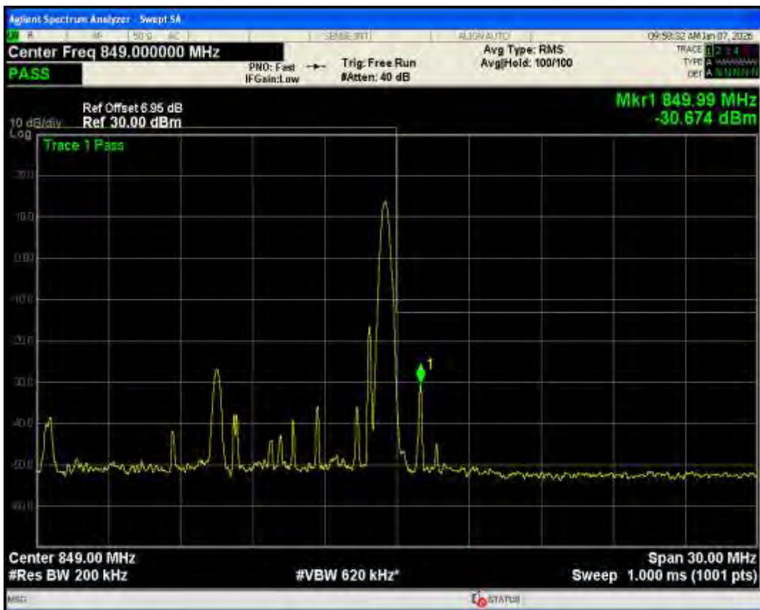
n26(824-849) SCS=15kHz CP QPSK BW=20MHz Channel=166800 RB=106@0
