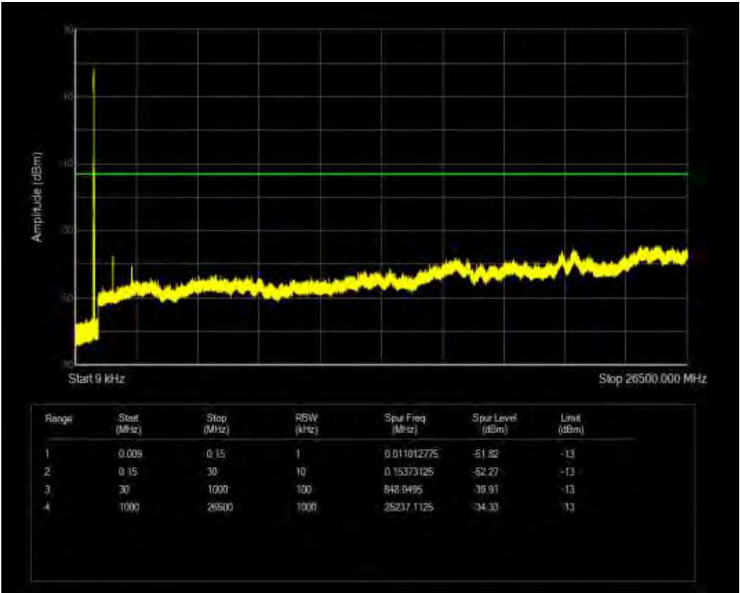
n26(814-824) SCS=15kHz CP QPSK BW=5MHz Channel=164300 RB=1@0
