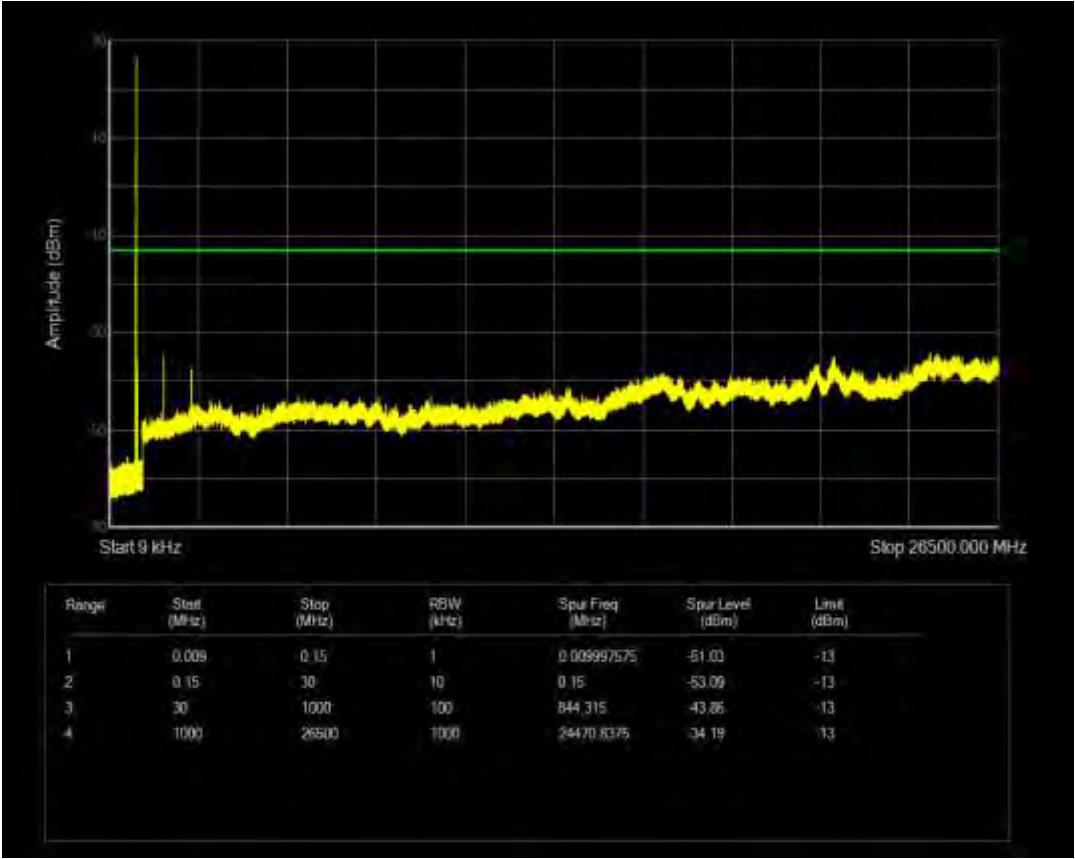
n26(814-824) SCS=15kHz CP QPSK BW=5MHz Channel=164300 RB=25@0
