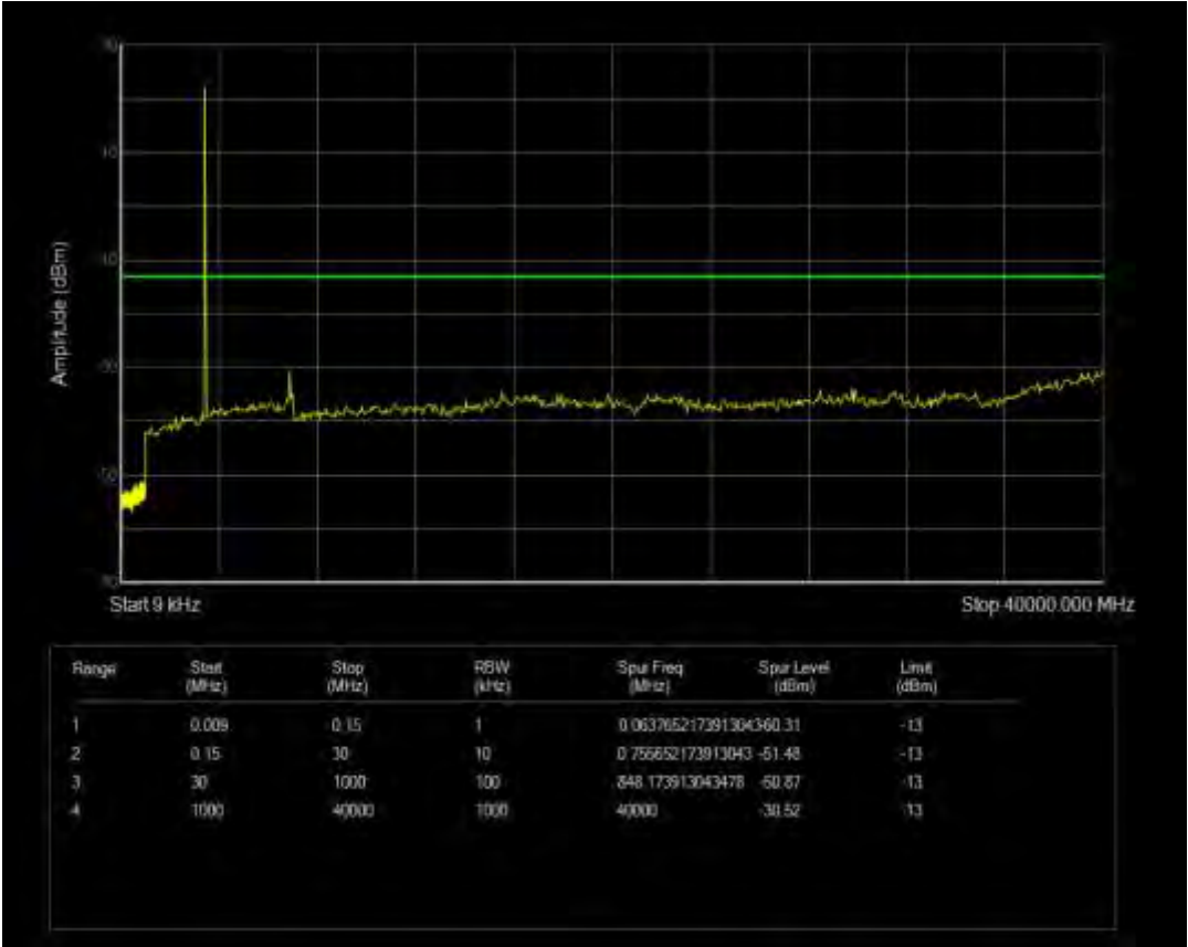
n78(3450-3550) SCS=30kHz CP QPSK BW=10MHz Channel=633334 RB=1@0
