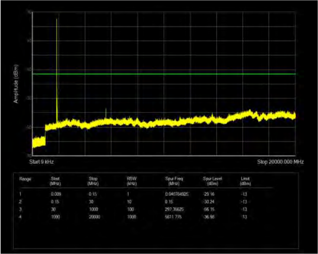
n2 SCS=15kHz CP QPSK BW=20MHz Channel=376000 RB=1@105
