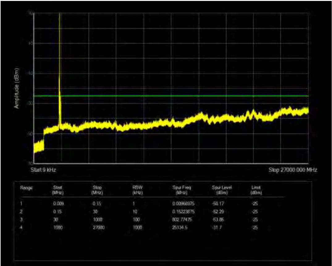
n41 SCS=30kHz CP QPSK BW=50MHz Channel=518598 RB=133@0
