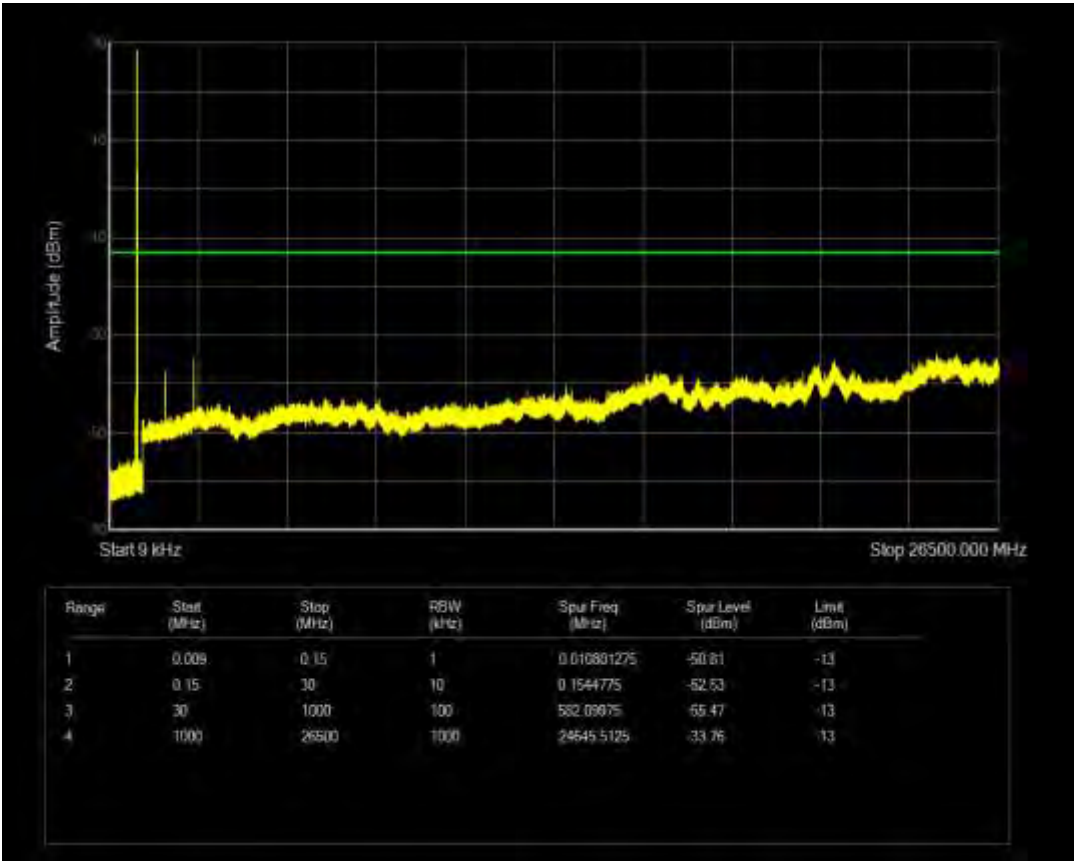
n26(824-849) SCS=15kHz CP QPSK BW=5MHz Channel=169300 RB=1@24
