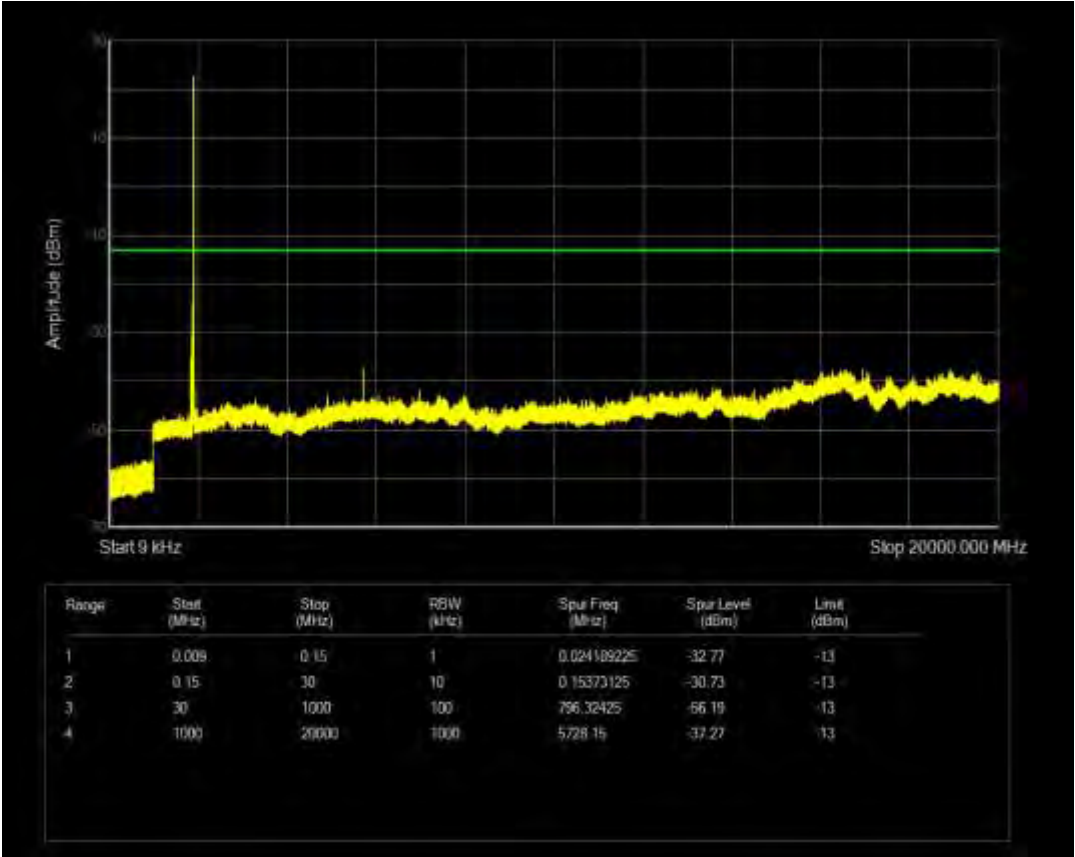
n2 SCS=15kHz CP QPSK BW=20MHz Channel=380000 RB=1@0
