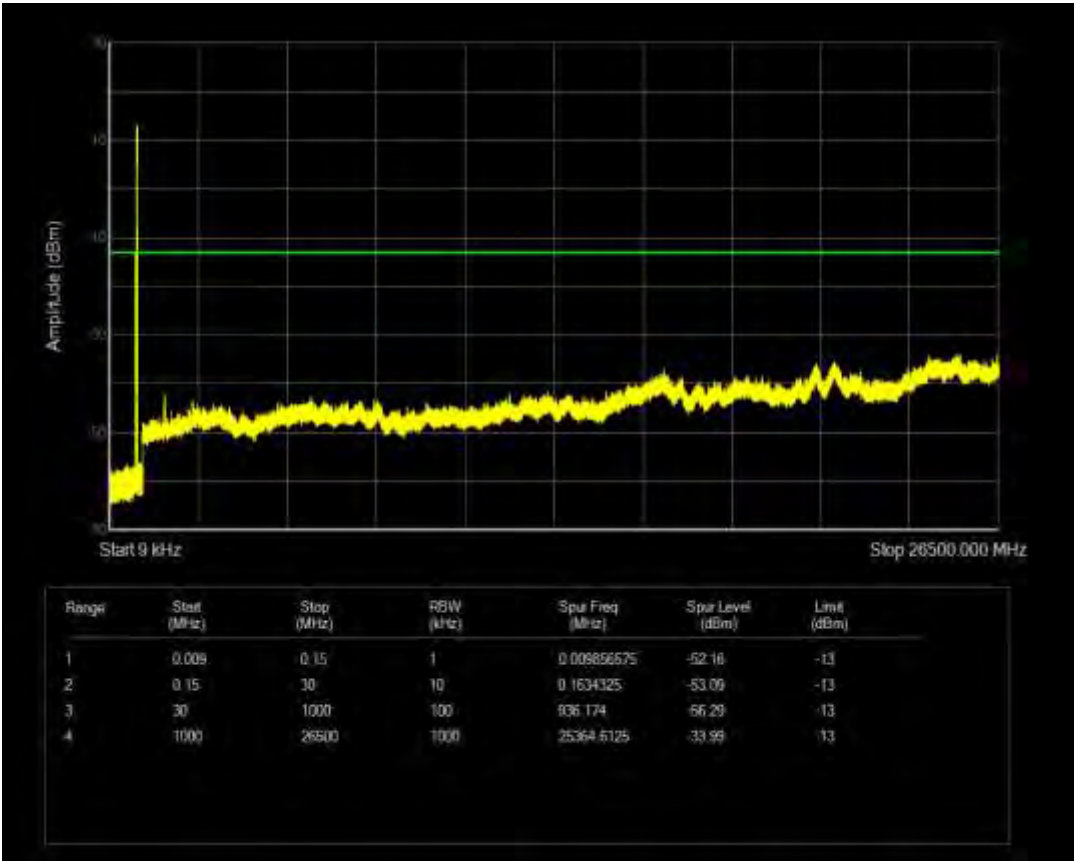
n26(824-849) SCS=15kHz CP QPSK BW=15MHz Channel=166300 RB=1@0
