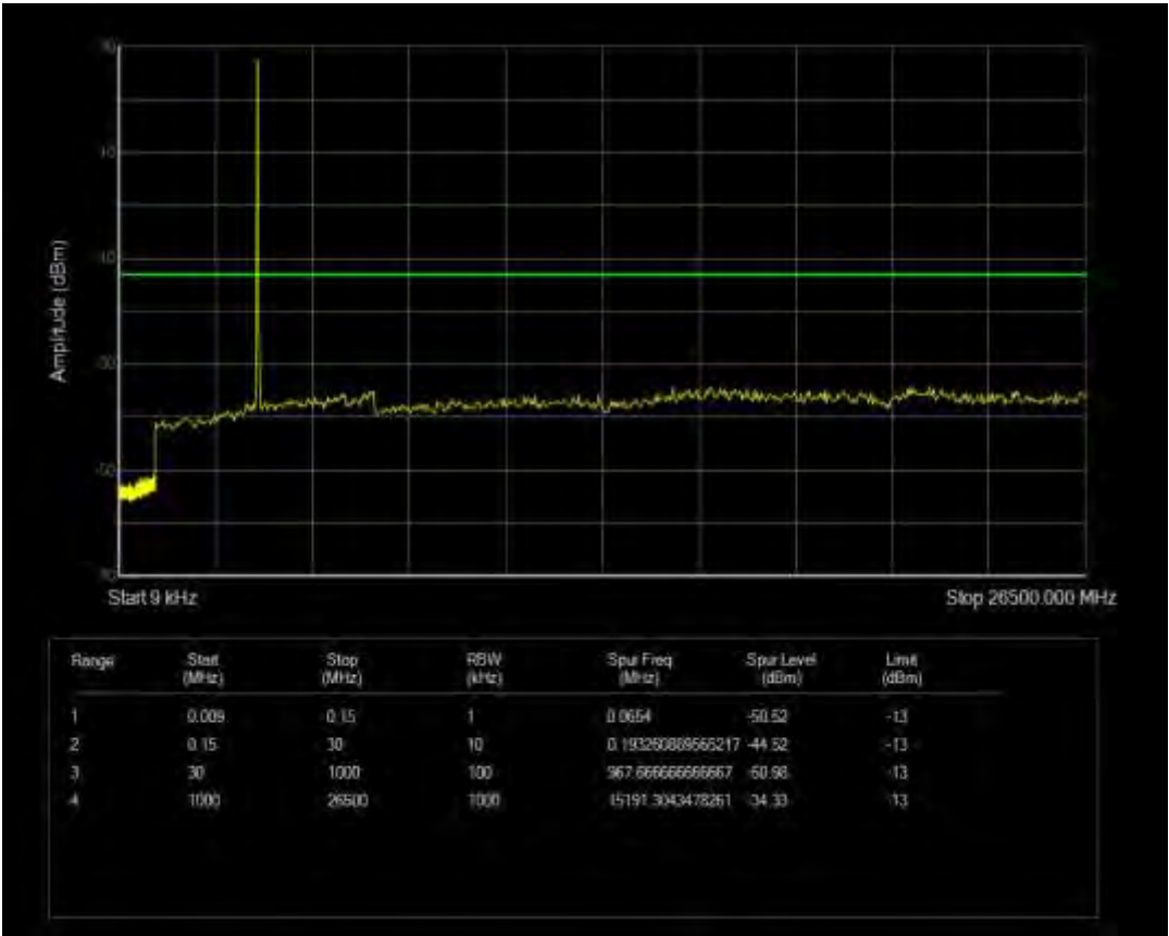
n77(3700-3980) SCS=30kHz CP QPSK BW=50MHz Channel=656000 RB=1@132
