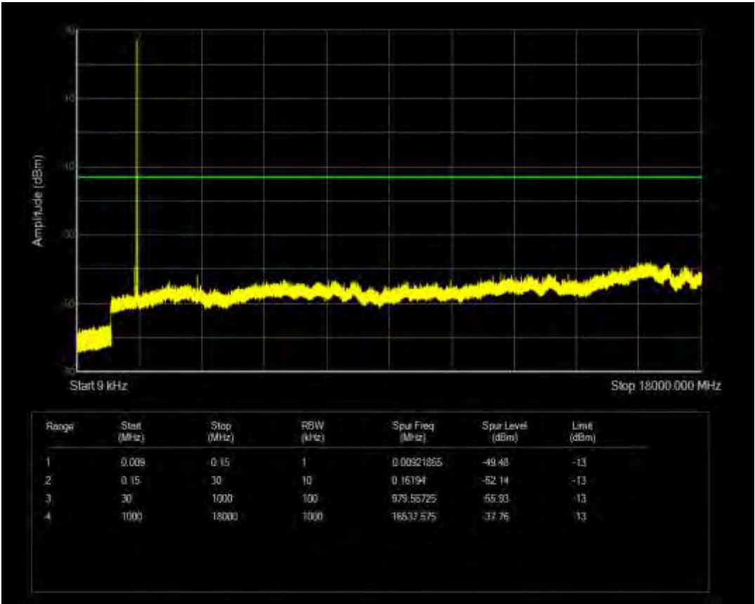
n66 SCS=15kHz CP QPSK BW=5MHz Channel=349000 RB=1@24
