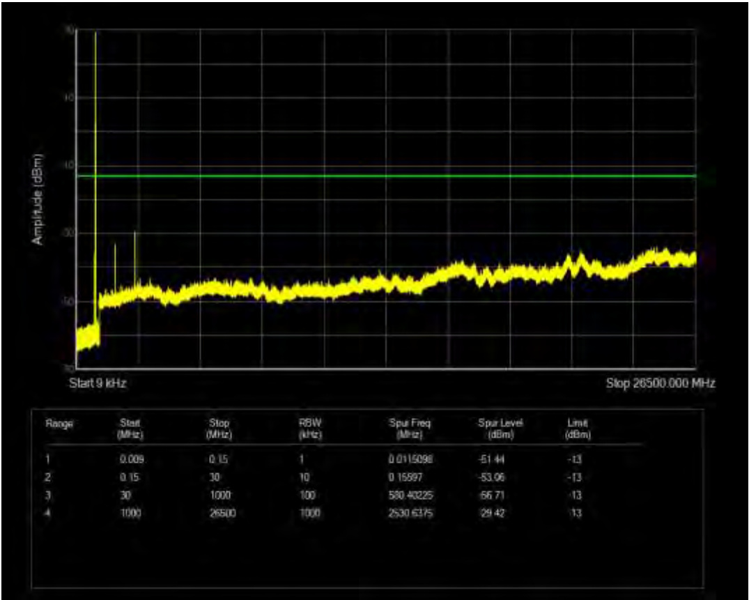
n26(824-849) SCS=15kHz CP QPSK BW=20MHz Channel=167800 RB=106@0
