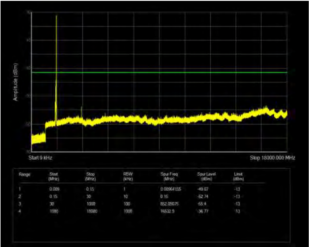
n66 SCS=15kHz CP QPSK BW=40MHz Channel=349000 RB=1@0
