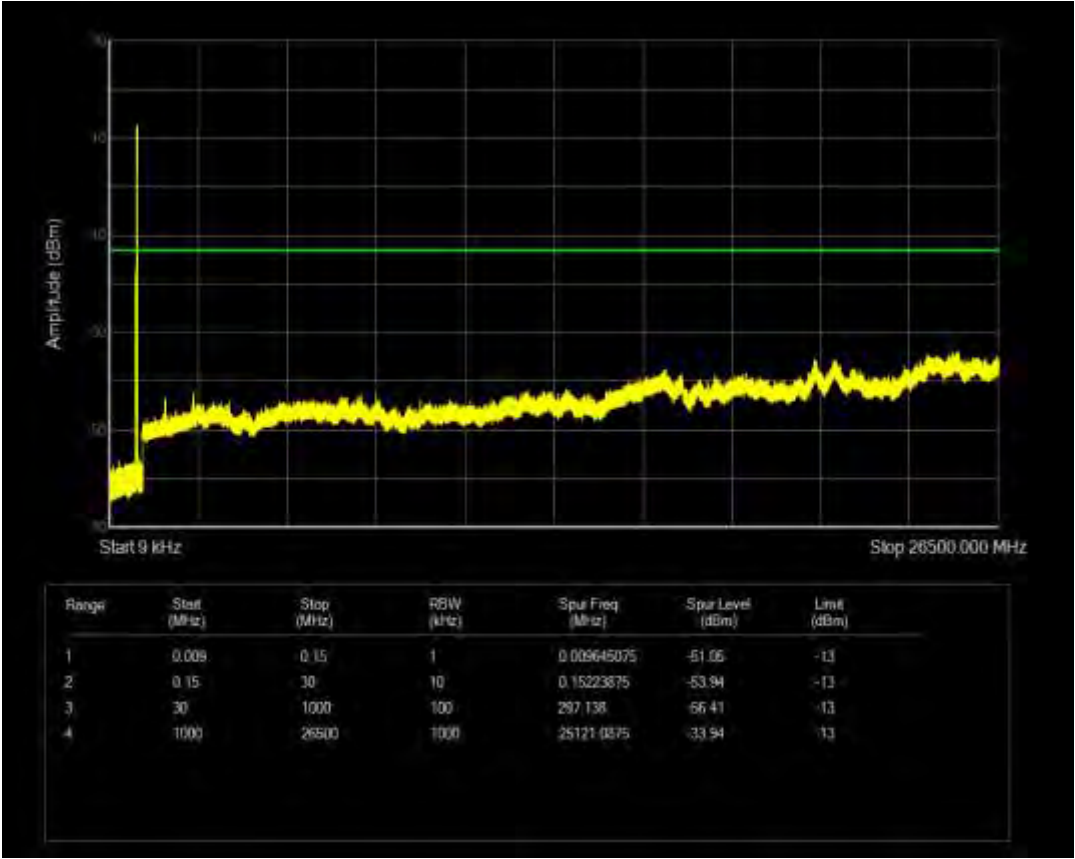
n26(824-849) SCS=15kHz CP QPSK BW=20MHz Channel=167800 RB=1@0
