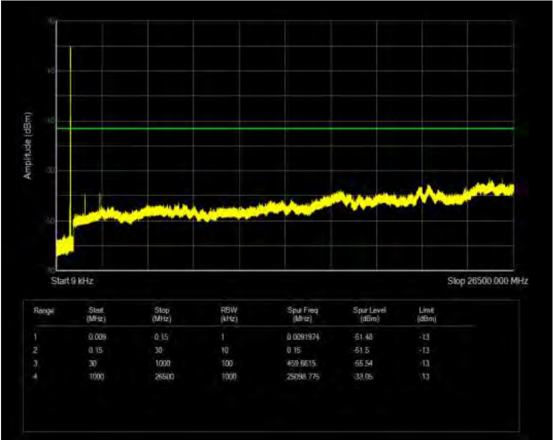
n26(824-849) SCS=15kHz CP QPSK BW=5MHz Channel=169300 RB=1@0
