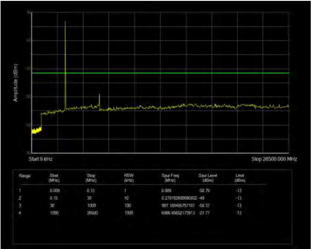
n77(3450-3550) SCS=30kHz CP QPSK BW=10MHz Channel=633334 RB=1@0
