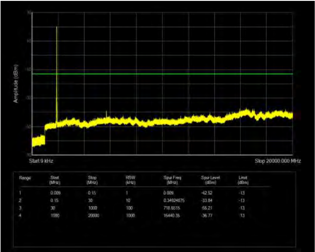
n26(814-824) SCS=15kHz CP QPSK BW=5MHz Channel=163300 RB=25@0
