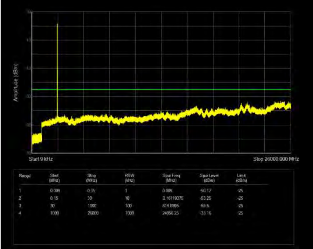
n77(3450-3550) SCS=30kHz CP QPSK BW=100MHz Channel=633332 RB=1@0
