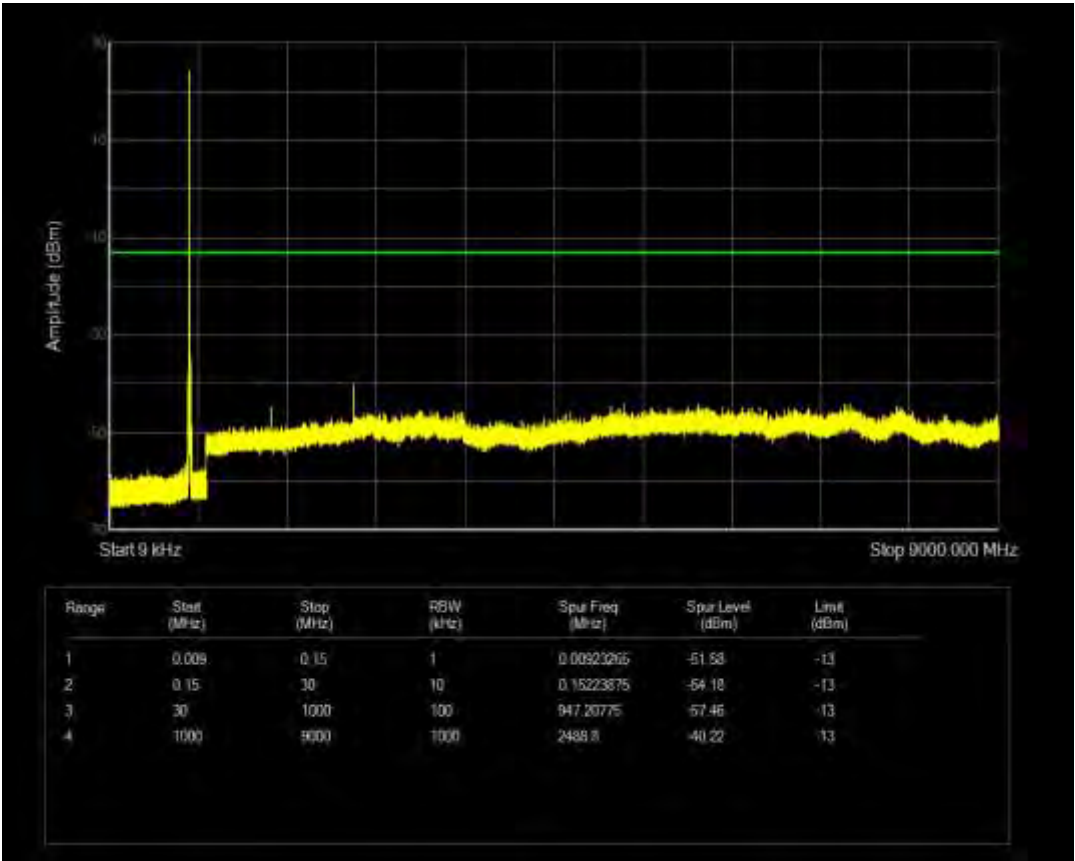
n5 SCS=15kHz CP QPSK BW=15MHz Channel=167300 RB=1@78
