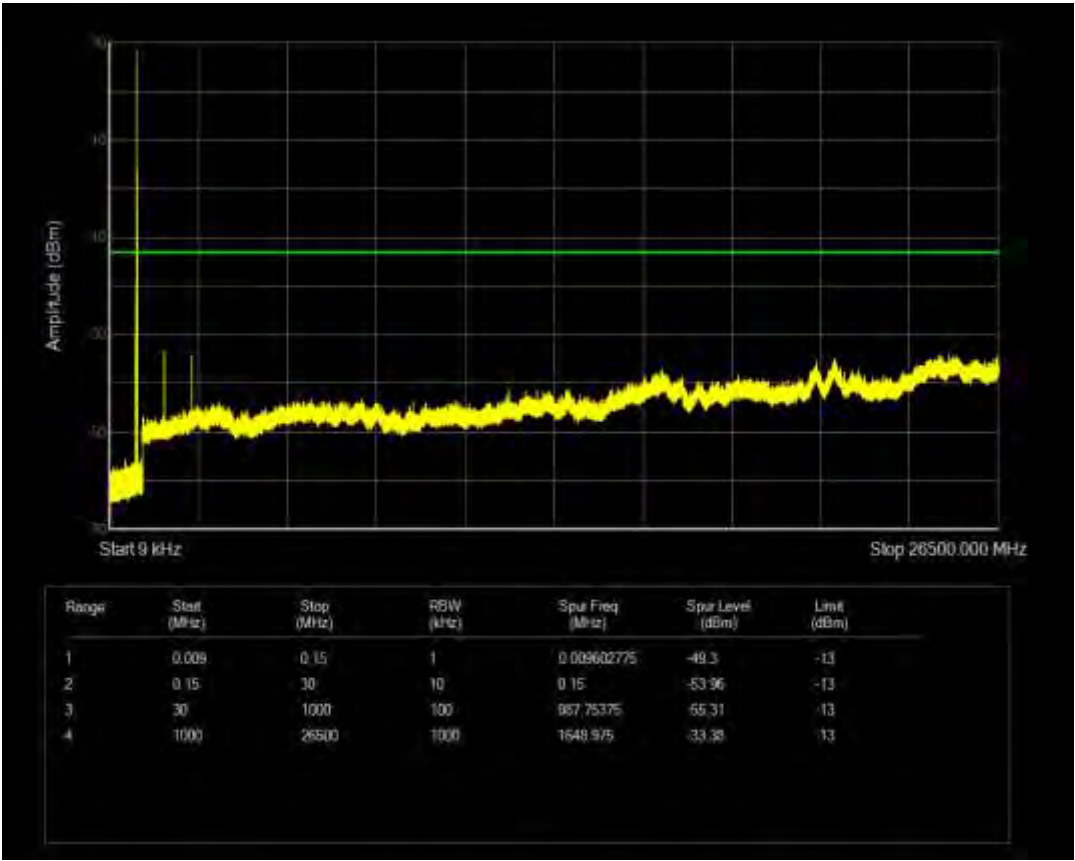
n26(824-849) SCS=15kHz CP QPSK BW=20MHz Channel=166800 RB=1@105
