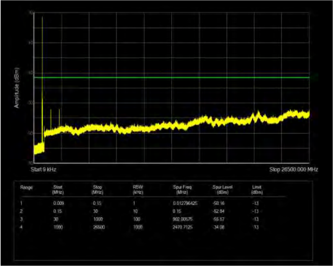
n26(824-849) SCS=15kHz CP QPSK BW=5MHz Channel=165300 RB=25@0
