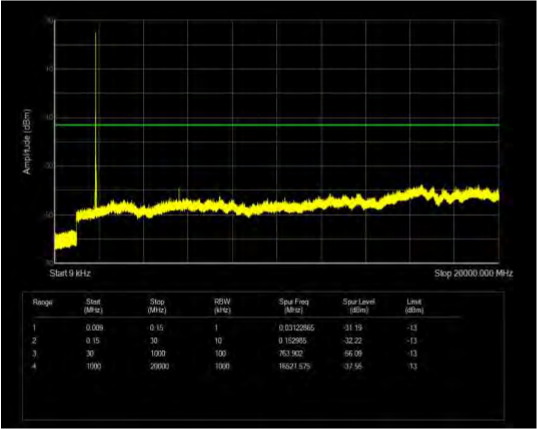
n2 SCS=15kHz CP QPSK BW=15MHz Channel=376000 RB=1@78
