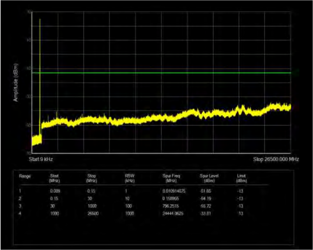
n26(824-849) SCS=15kHz CP QPSK BW=15MHz Channel=166300 RB=79@0
