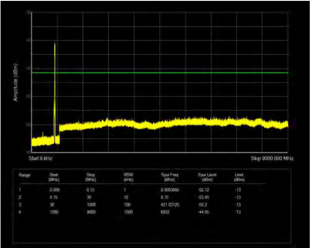
n5 SCS=15kHz CP QPSK BW=20MHz Channel=167300 RB=1@0
