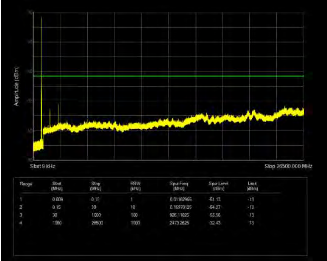
n26(824-849) SCS=15kHz CP QPSK BW=5MHz Channel=165300 RB=1@24
