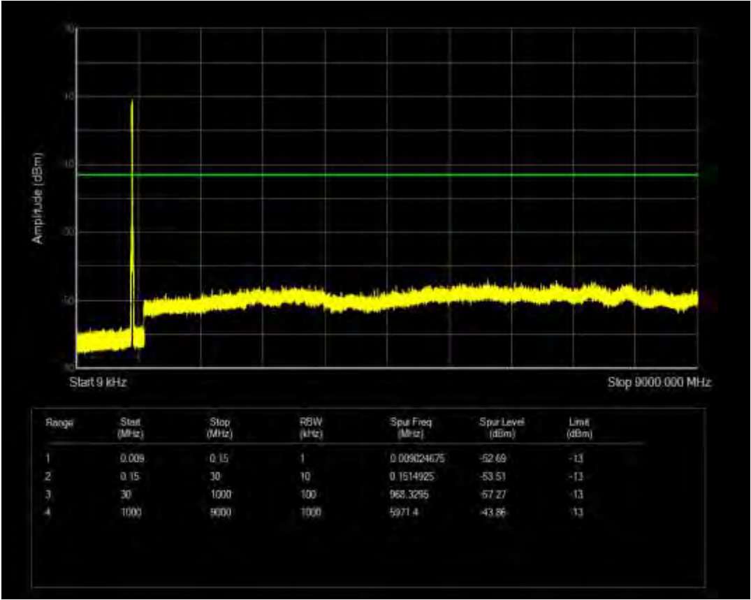
n5 SCS=15kHz CP QPSK BW=15MHz Channel=167300 RB=1@0
