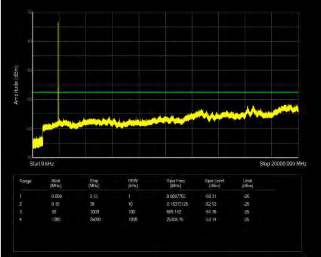
n7 SCS=15kHz CP QPSK BW=5MHz Channel=507000 RB=1@0
