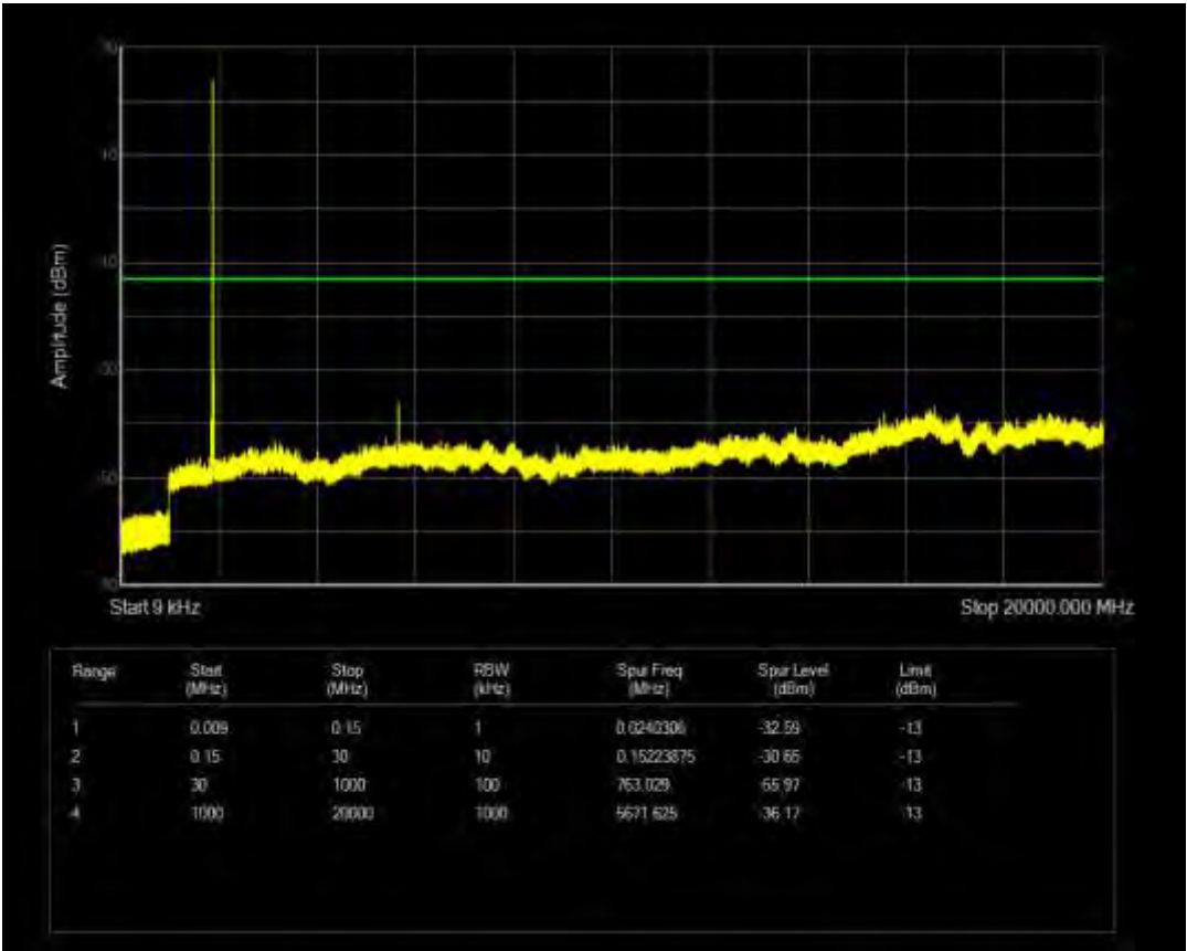
n2 SCS=15kHz CP QPSK BW=20MHz Channel=376000 RB=1@0
