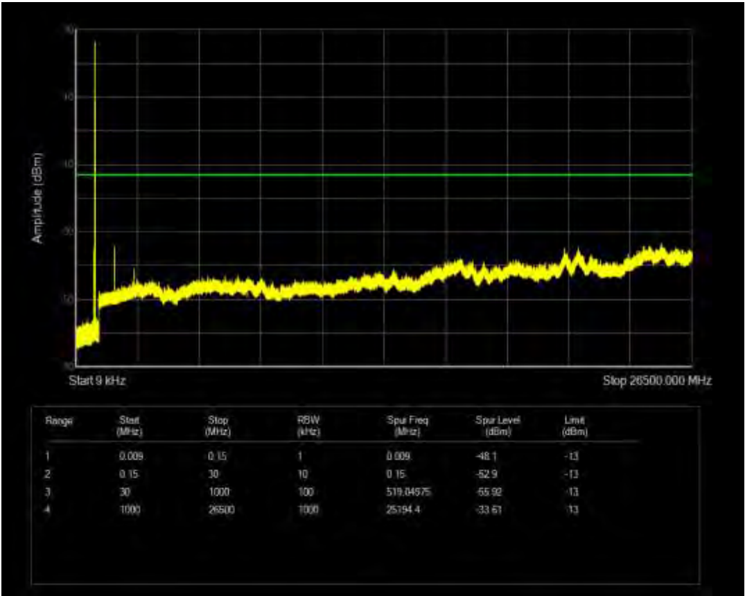
n26(824-849) SCS=15kHz CP QPSK BW=15MHz Channel=168300 RB=79@0
