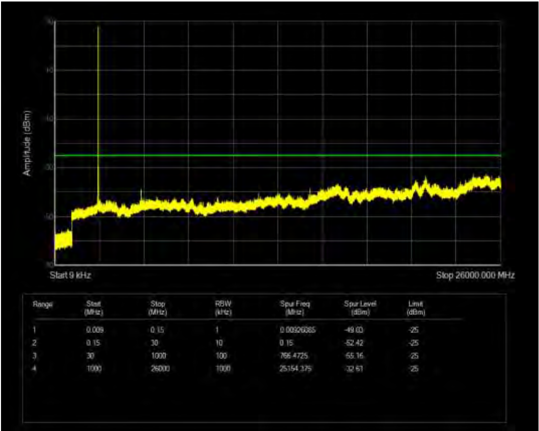
n7 SCS=15kHz CP QPSK BW=20MHz Channel=507000 RB=1@105
