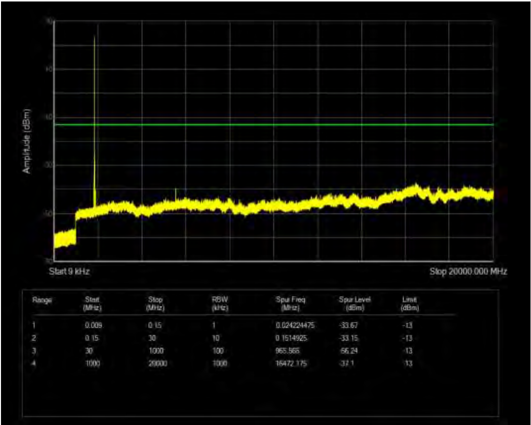
n2 SCS=15kHz CP QPSK BW=15MHz Channel=371500 RB=1@78
