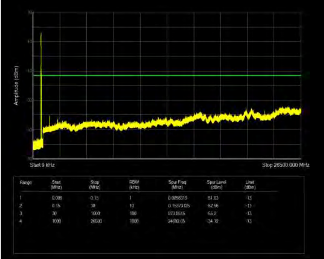
n26(814-824) SCS=15kHz CP QPSK BW=10MHz Channel=163800 RB=1@0
