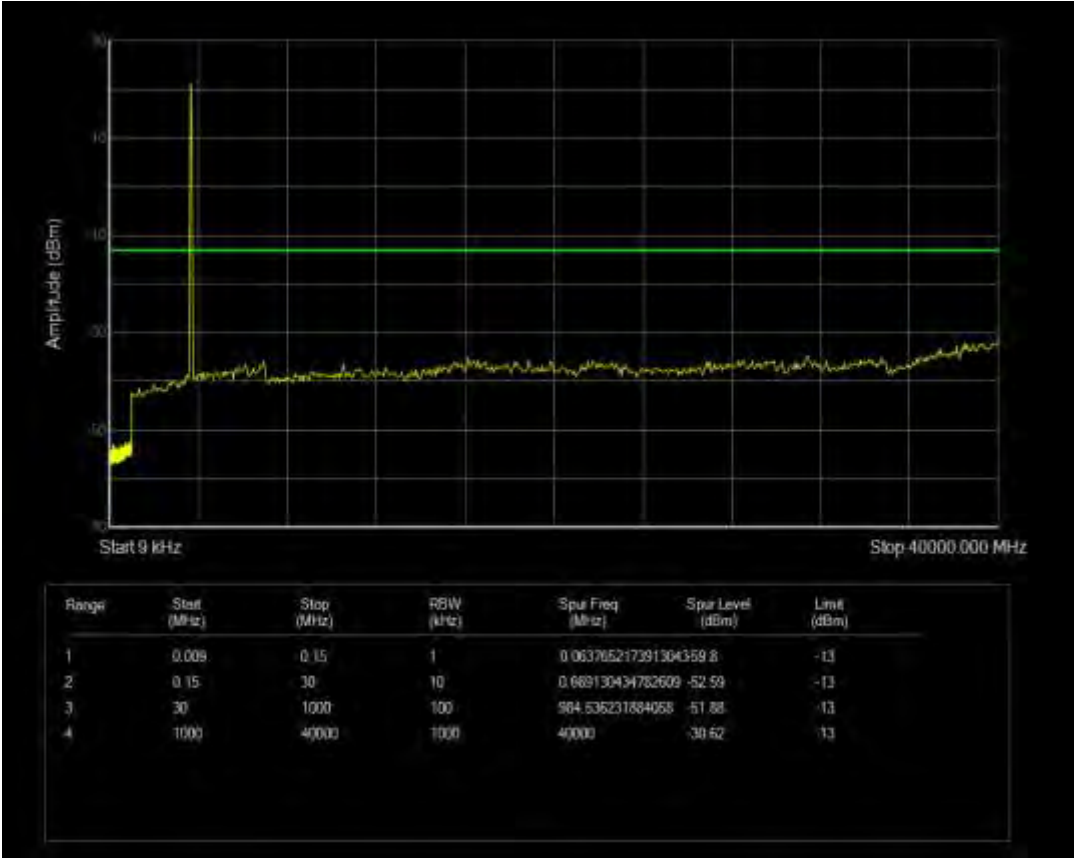
n77(3700-3980) SCS=30kHz CP QPSK BW=10MHz Channel=656000 RB=1@0
