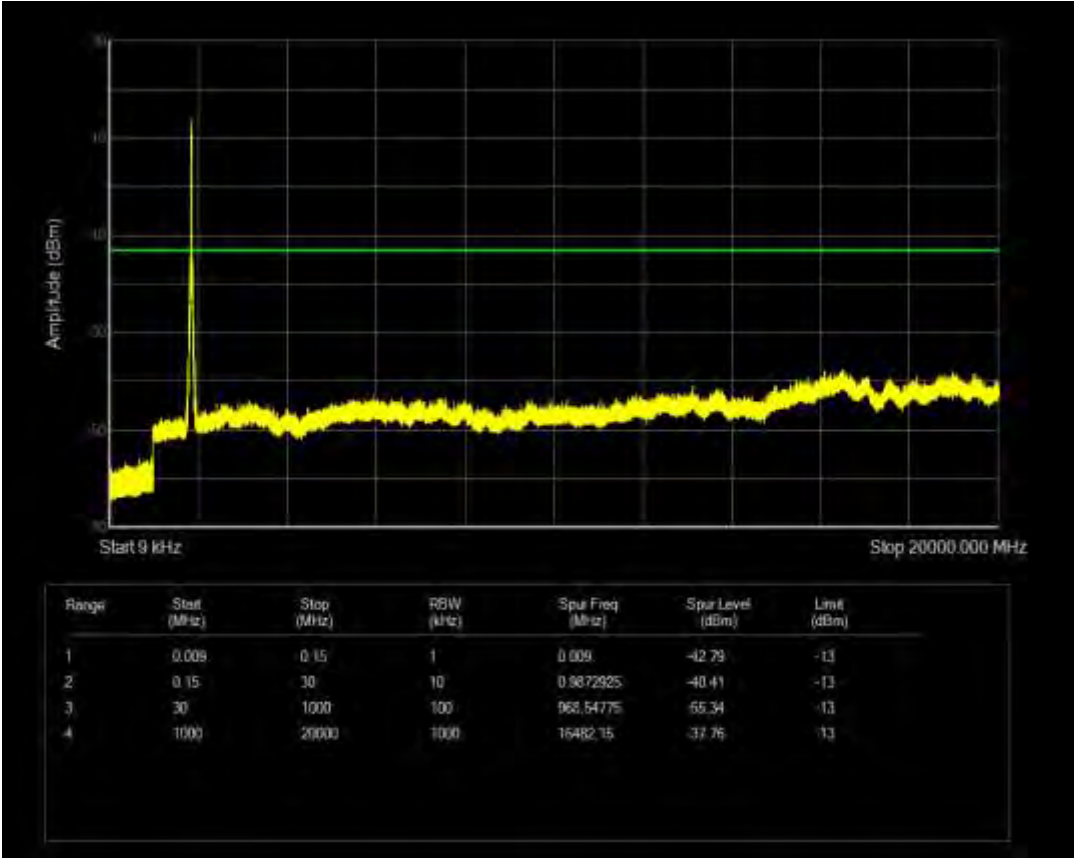
n2 SCS=15kHz CP QPSK BW=20MHz Channel=372000 RB=1@0
