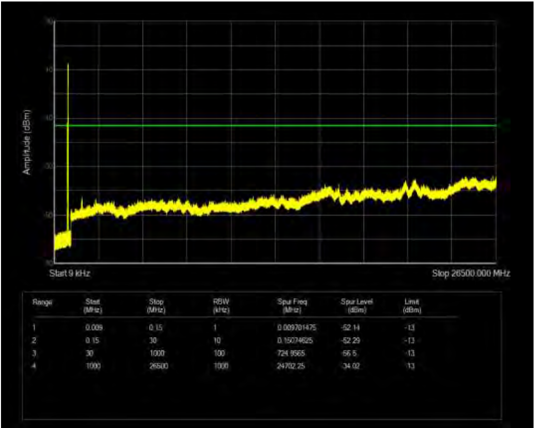
n26(824-849) SCS=15kHz CP QPSK BW=20MHz Channel=166800 RB=1@0
