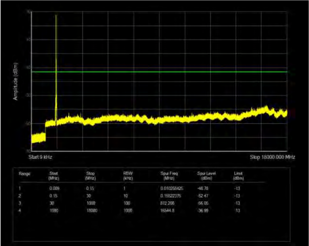
n66 SCS=15kHz CP QPSK BW=40MHz Channel=349000 RB=1@215
