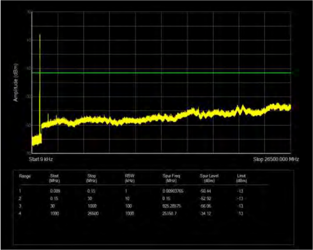
n26(824-849) SCS=15kHz CP QPSK BW=15MHz Channel=168300 RB=1@0
