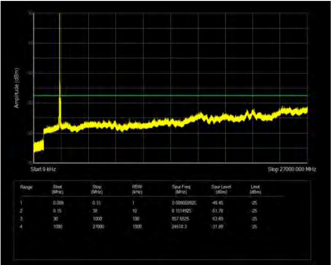
n41 SCS=30kHz CP QPSK BW=50MHz Channel=518598 RB=1@132
