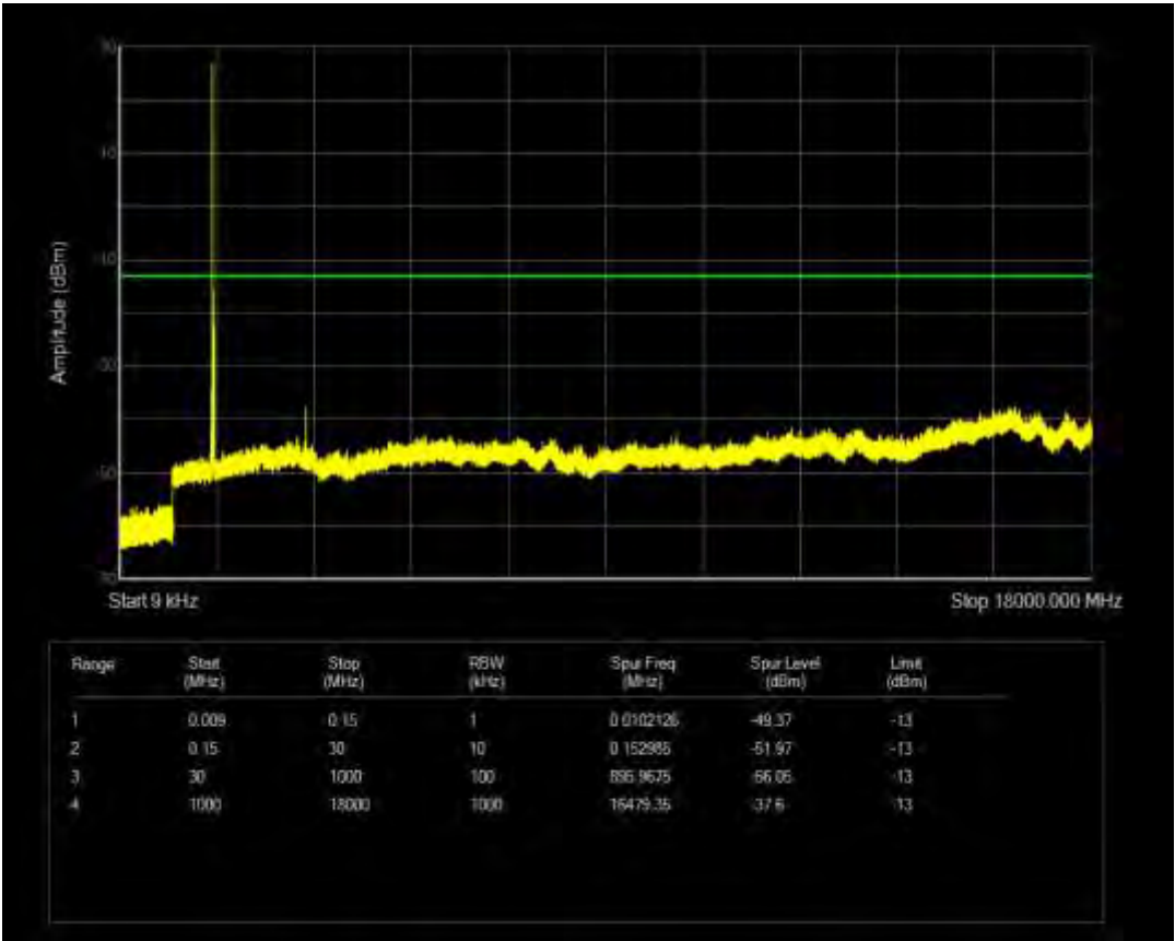
n66 SCS=15kHz CP QPSK BW=20MHz Channel=349000 RB=1@105
