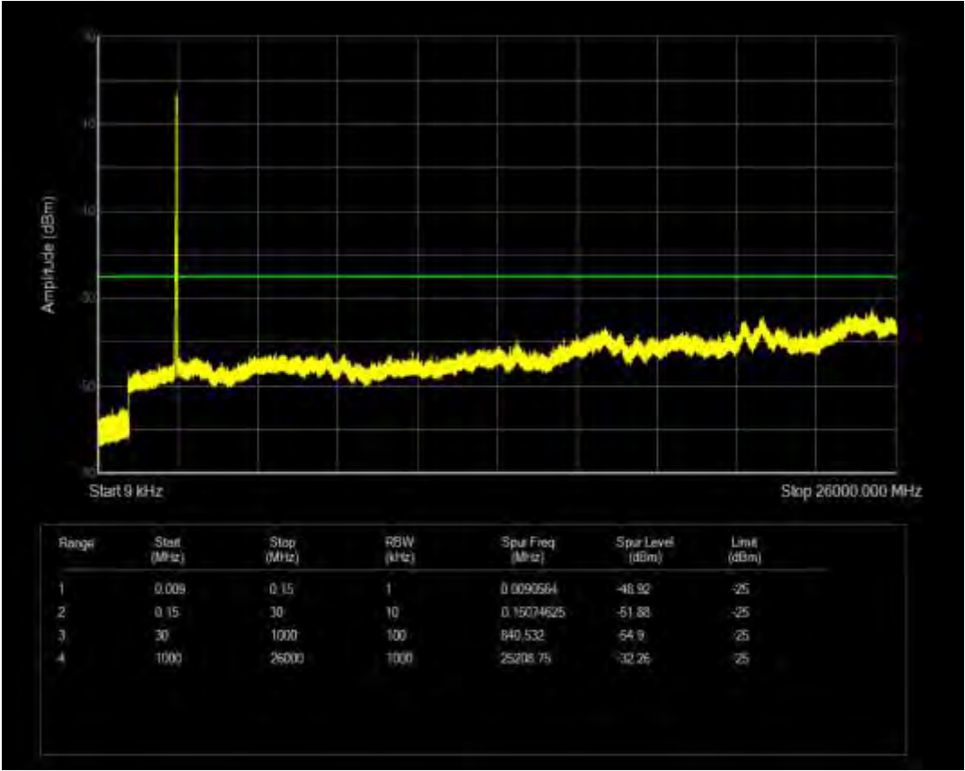
n7 SCS=15kHz CP QPSK BW=20MHz Channel=507000 RB=1@0
