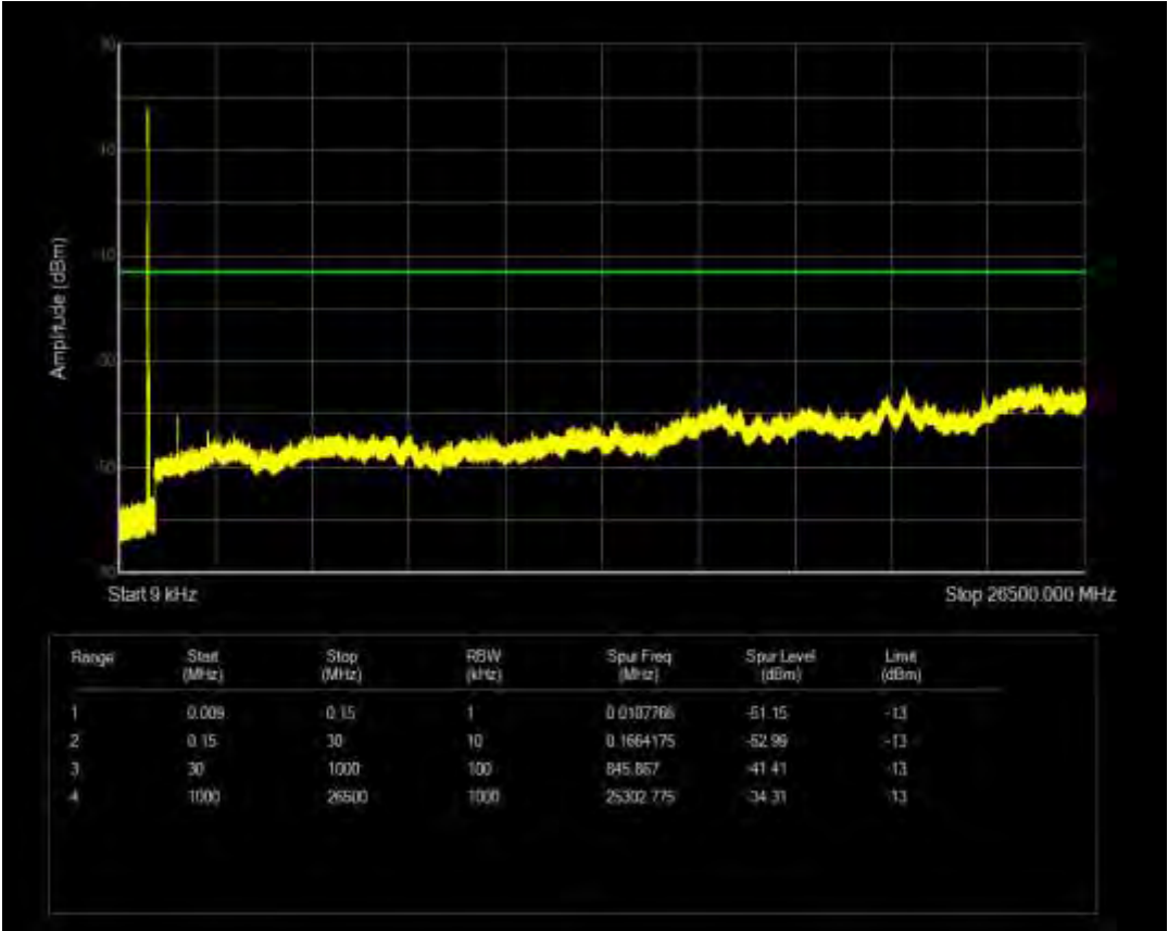
n26(814-824) SCS=15kHz CP QPSK BW=5MHz Channel=163300 RB=1@0
