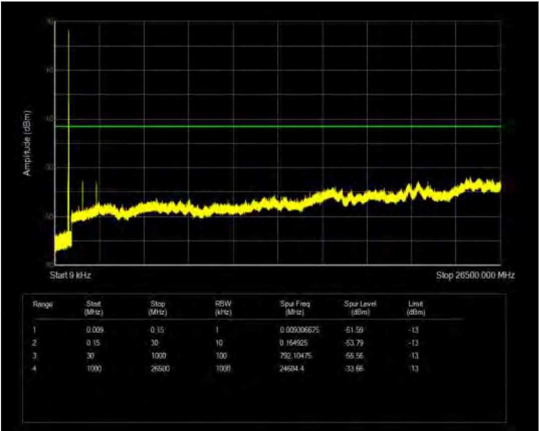
n26(824-849) SCS=15kHz CP QPSK BW=5MHz Channel=169300 RB=25@0
