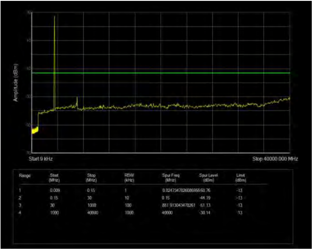
n78(3450-3550) SCS=30kHz CP QPSK BW=10MHz Channel=633334 RB=24@0
