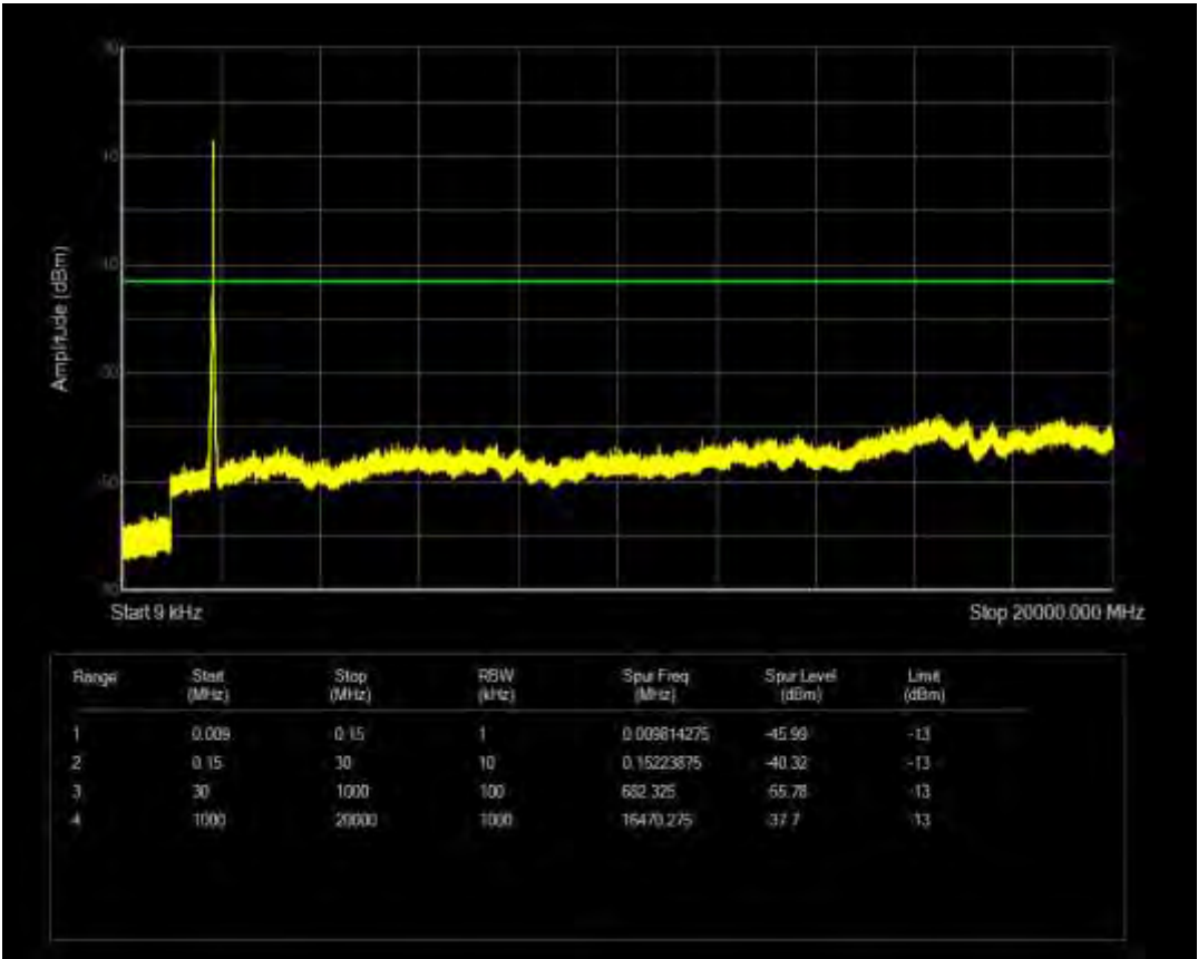
n2 SCS=15kHz CP QPSK BW=15MHz Channel=376000 RB=1@0
