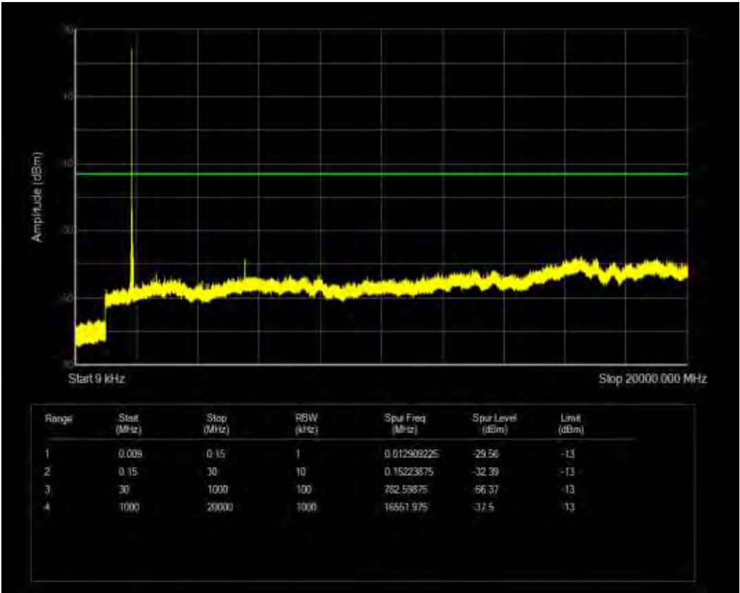
n2 SCS=15kHz CP QPSK BW=20MHz Channel=372000 RB=1@105
