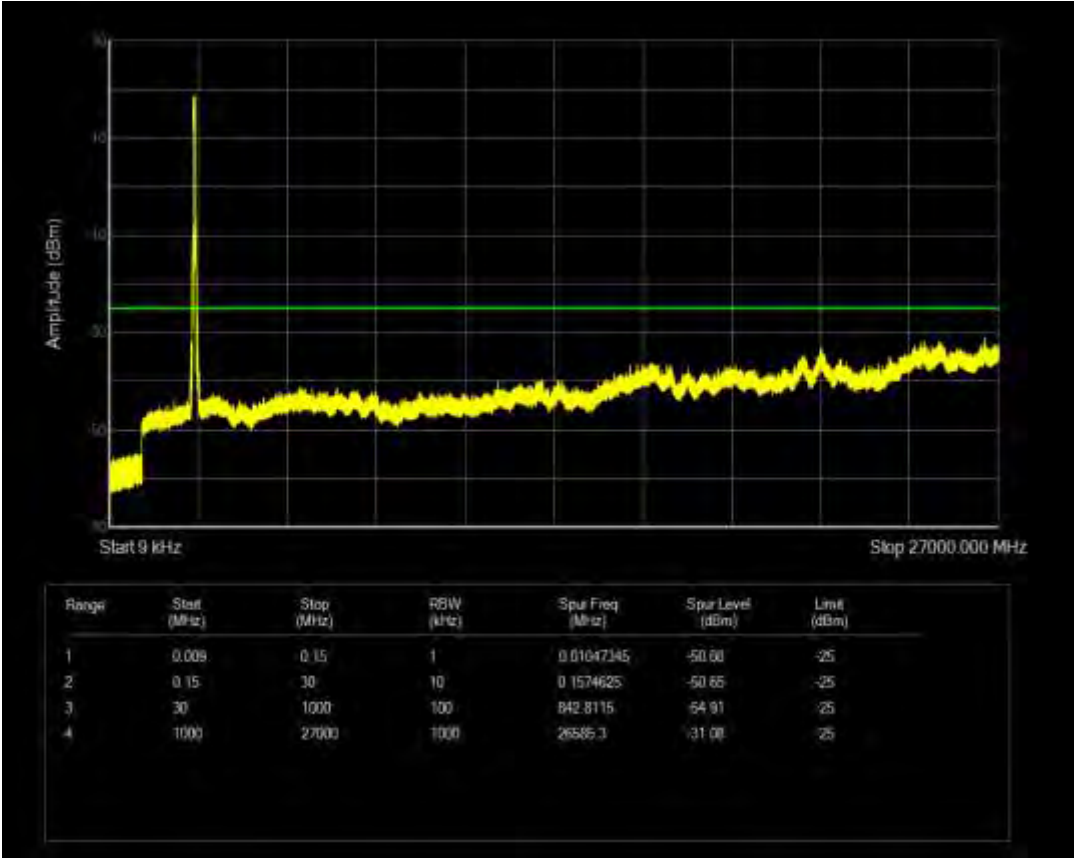
n41 SCS=30kHz CP QPSK BW=50MHz Channel=518598 RB=1@0
