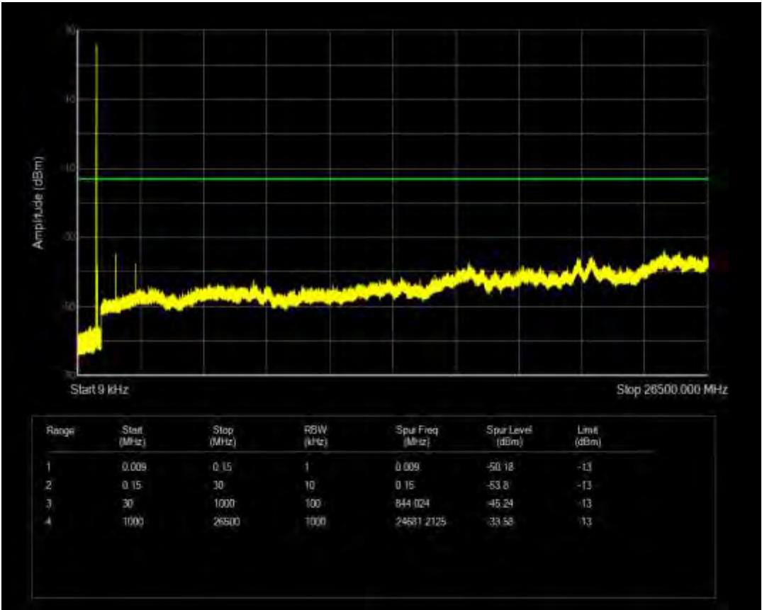
n26(814-824) SCS=15kHz CP QPSK BW=5MHz Channel=163300 RB=1@24
