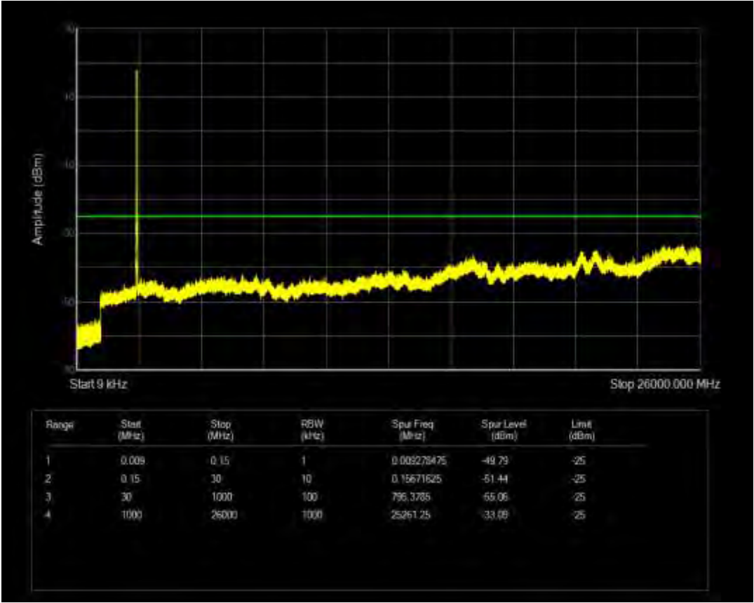
n7 SCS=15kHz CP QPSK BW=15MHz Channel=507000 RB=1@0
