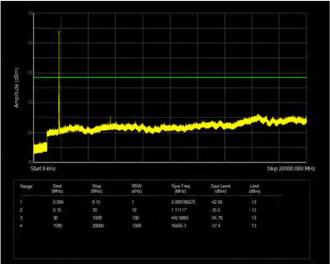
n2 SCS=15kHz CP QPSK BW=5MHz Channel=381500 RB=1@0
