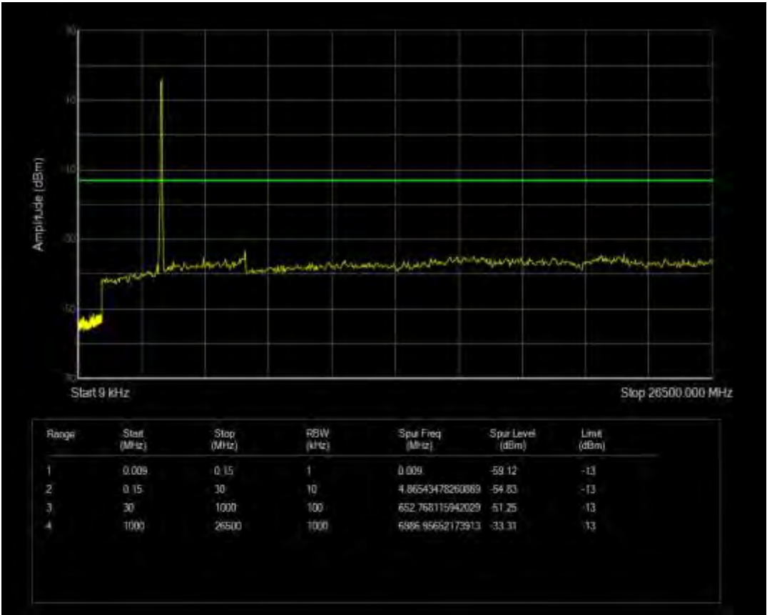
n77(3450-3550) SCS=30kHz CP QPSK BW=50MHz Channel=633334 RB=1@0
