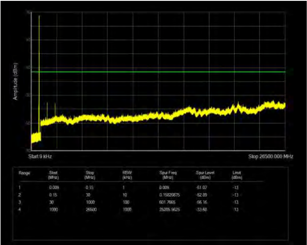
n26(824-849) SCS=15kHz CP QPSK BW=15MHz Channel=168300 RB=1@78
