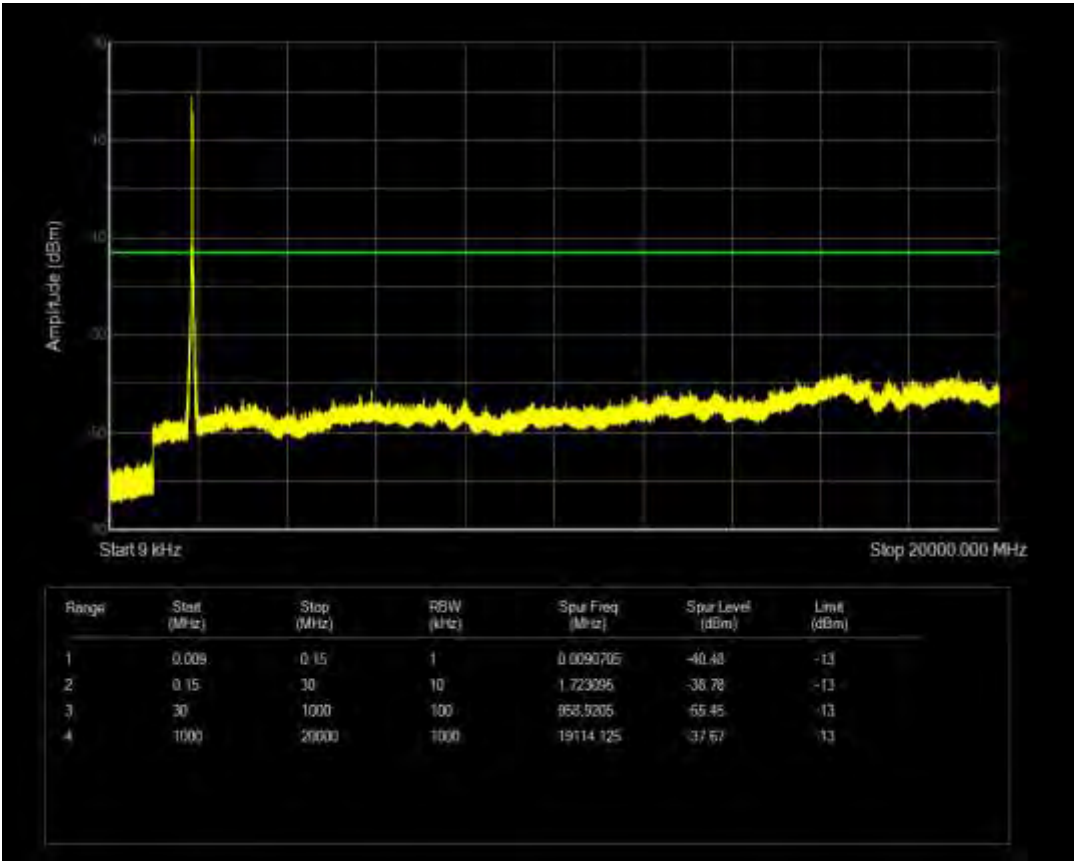
n2 SCS=15kHz CP QPSK BW=20MHz Channel=380000 RB=1@105
