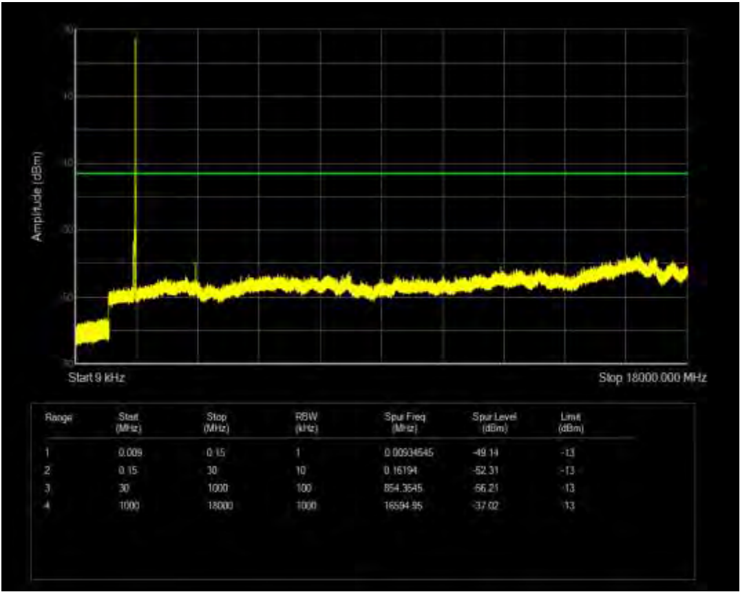
n66 SCS=15kHz CP QPSK BW=5MHz Channel=349000 RB=1@0
