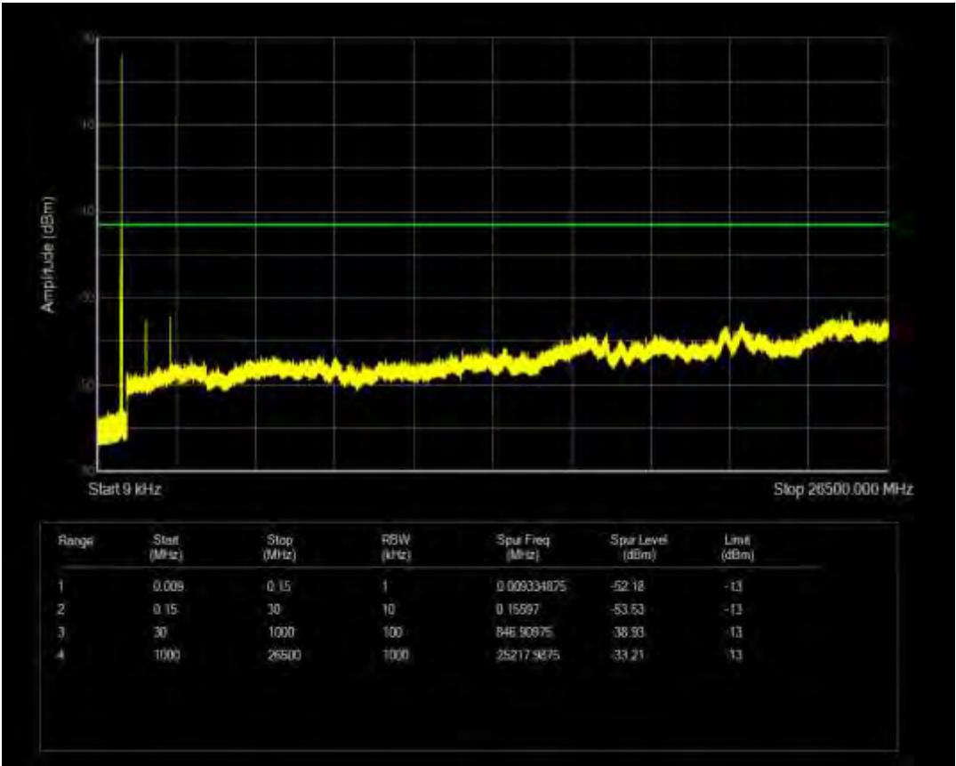
n26(814-824) SCS=15kHz CP QPSK BW=10MHz Channel=163800 RB=52@0
