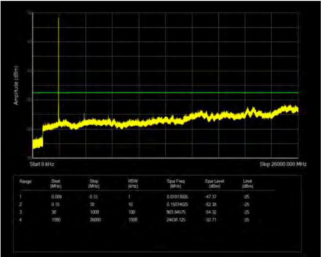
n7 SCS=15kHz CP QPSK BW=15MHz Channel=507000 RB=1@78
