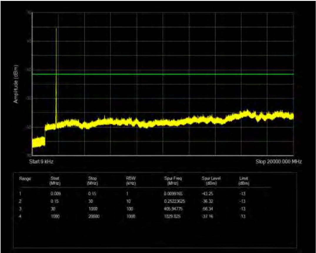
n2 SCS=15kHz CP QPSK BW=5MHz Channel=376000 RB=1@0
