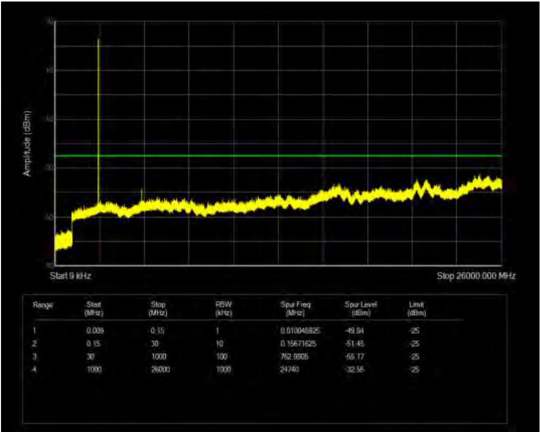
n7 SCS=15kHz CP QPSK BW=5MHz Channel=507000 RB=1@24
