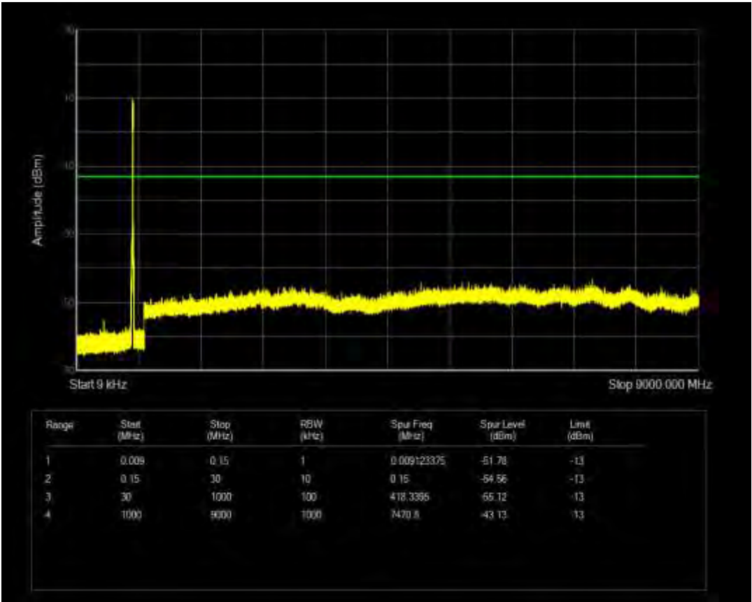
n5 SCS=15kHz CP QPSK BW=15MHz Channel=168300 RB=1@0
