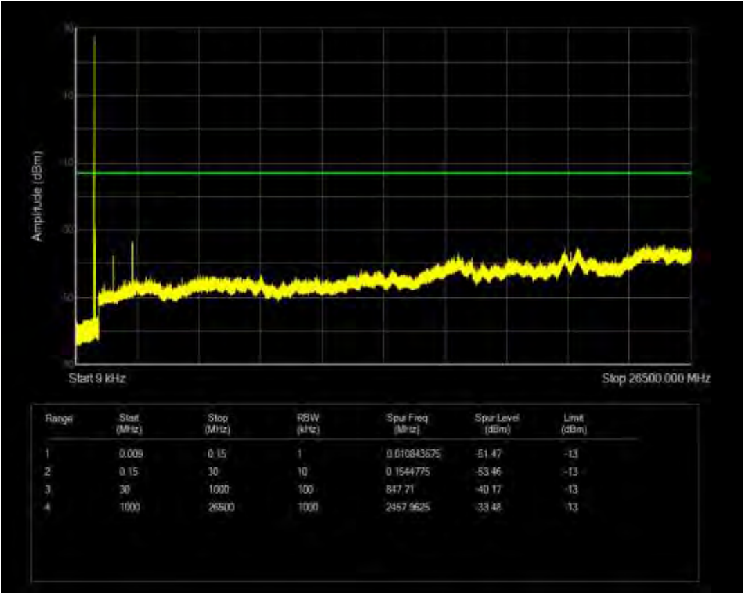
n26(814-824) SCS=15kHz CP QPSK BW=5MHz Channel=164300 RB=1@24
