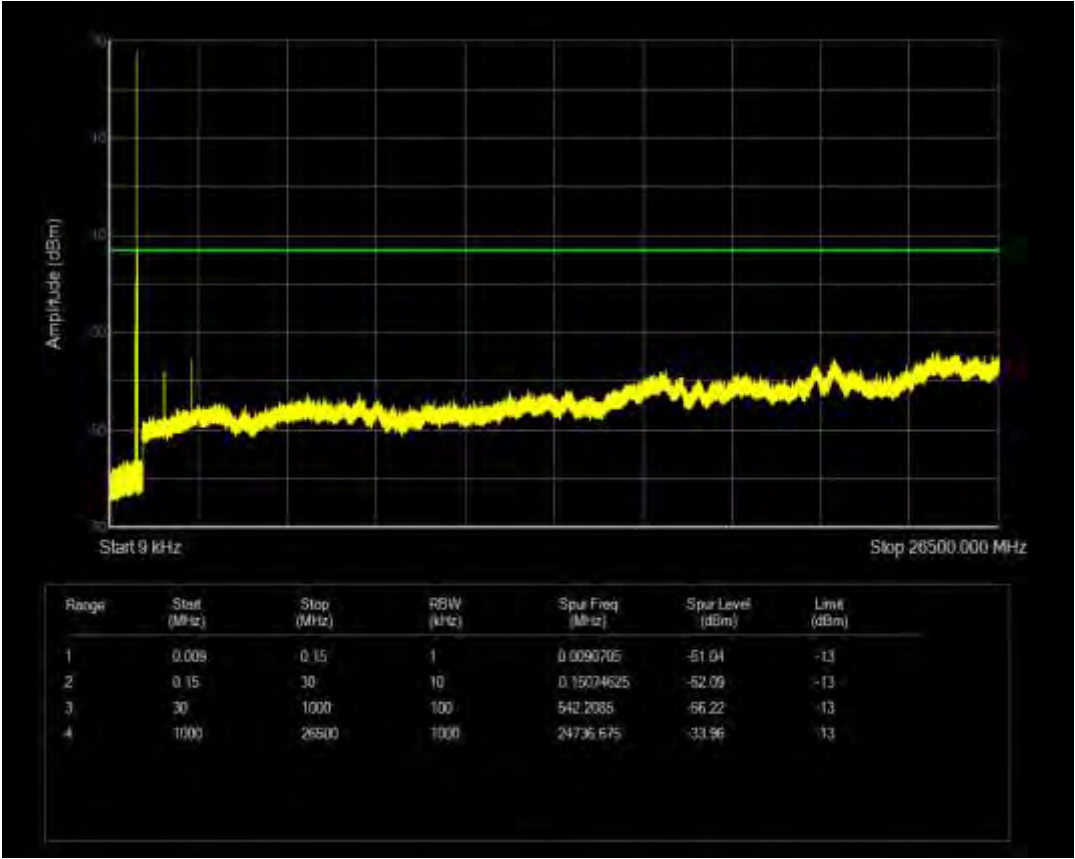
n26(824-849) SCS=15kHz CP QPSK BW=15MHz Channel=166300 RB=1@78
