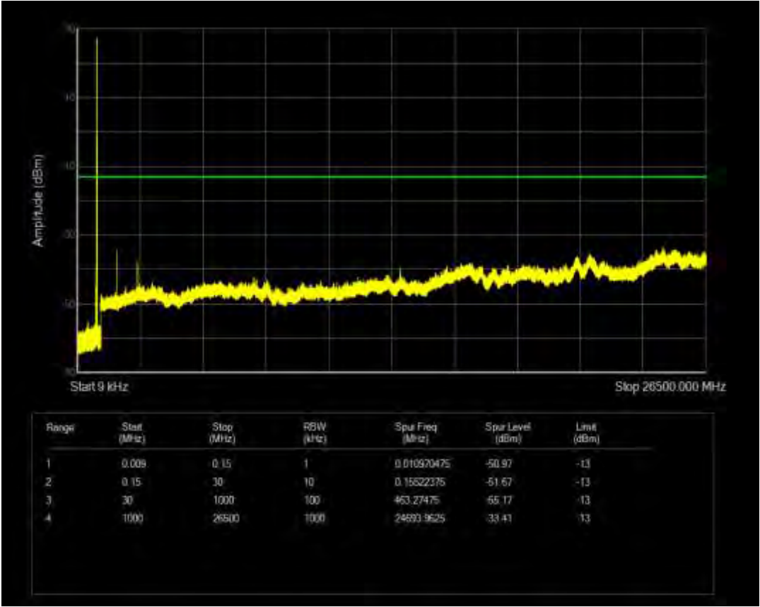
n26(824-849) SCS=15kHz CP QPSK BW=20MHz Channel=166800 RB=106@0
