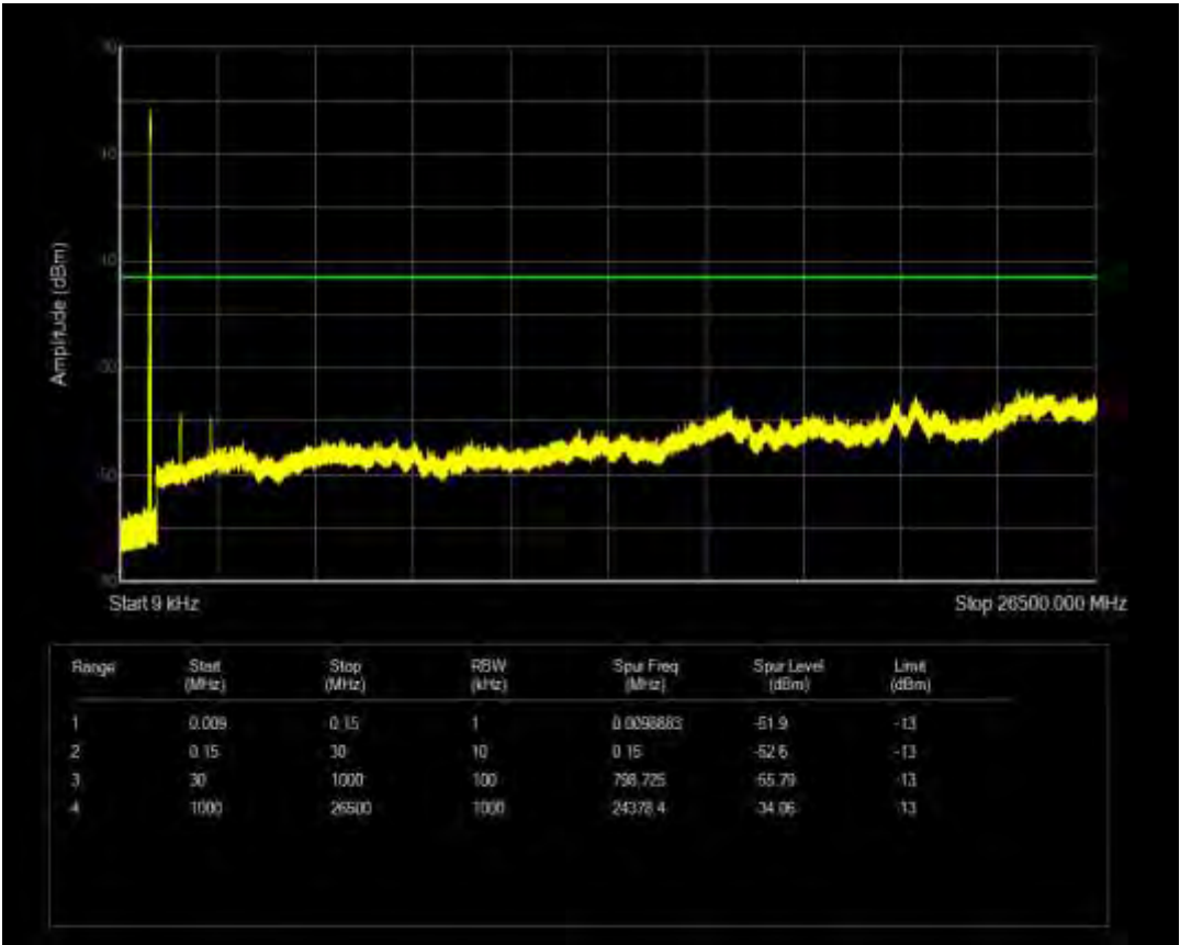
n26(824-849) SCS=15kHz CP QPSK BW=5MHz Channel=165300 RB=1@0
