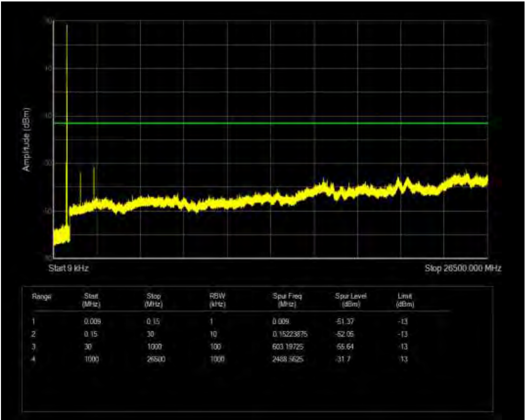
n26(824-849) SCS=15kHz CP QPSK BW=20MHz Channel=167800 RB=1@105
