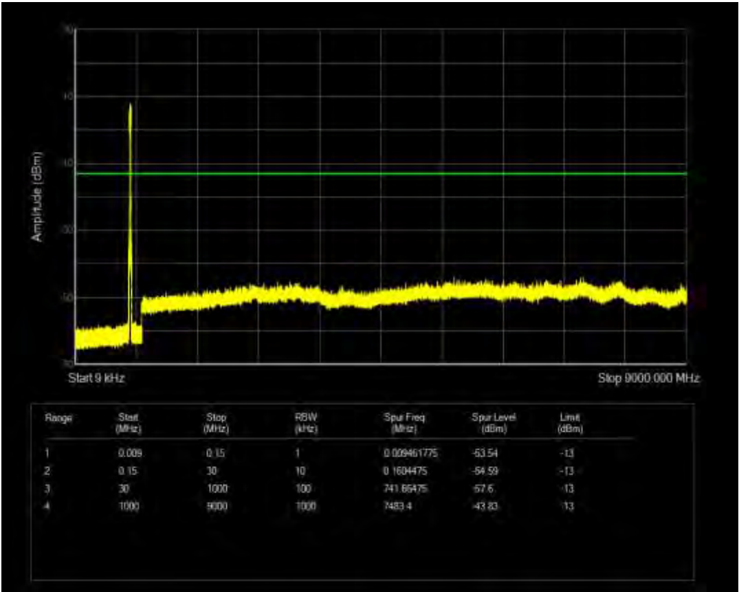
n5 SCS=15kHz CP QPSK BW=20MHz Channel=167300 RB=1@105
