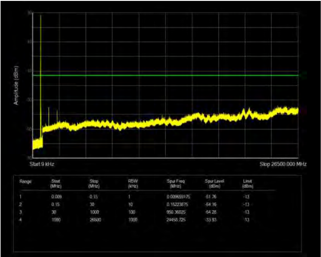
n26(814-824) SCS=15kHz CP QPSK BW=10MHz Channel=163800 RB=1@51
