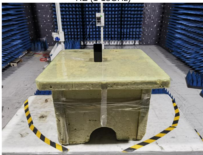
RE (1-18GHz)
