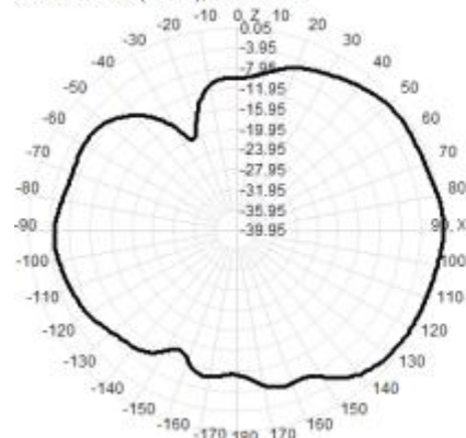
2450.0MHz Total(E1-XZ), Max= 0.05dBi
