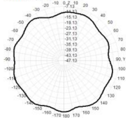
950.0MHz Total(E2-YZ), Max=-8.74dBi
