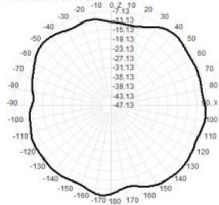
950.0MHz Total(E1-XZ), Max=-7.13dBi
