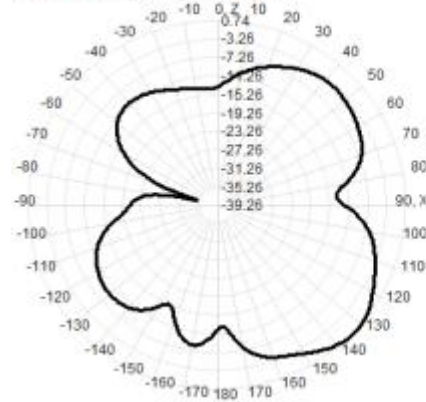
2100.0MHz Total(E1-XZ), Max= 0.74dBi
