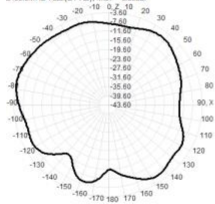
2400.0MHz Total(E1-XZ), Max= -3.60dBi
