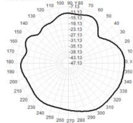
Total(H-XY), Max=-8.16dBi, CirD=10.68
