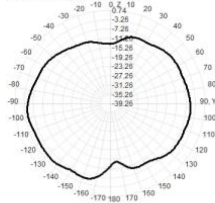
2100.0MHz Total(E2-YZ), Max= -4.57dBi
