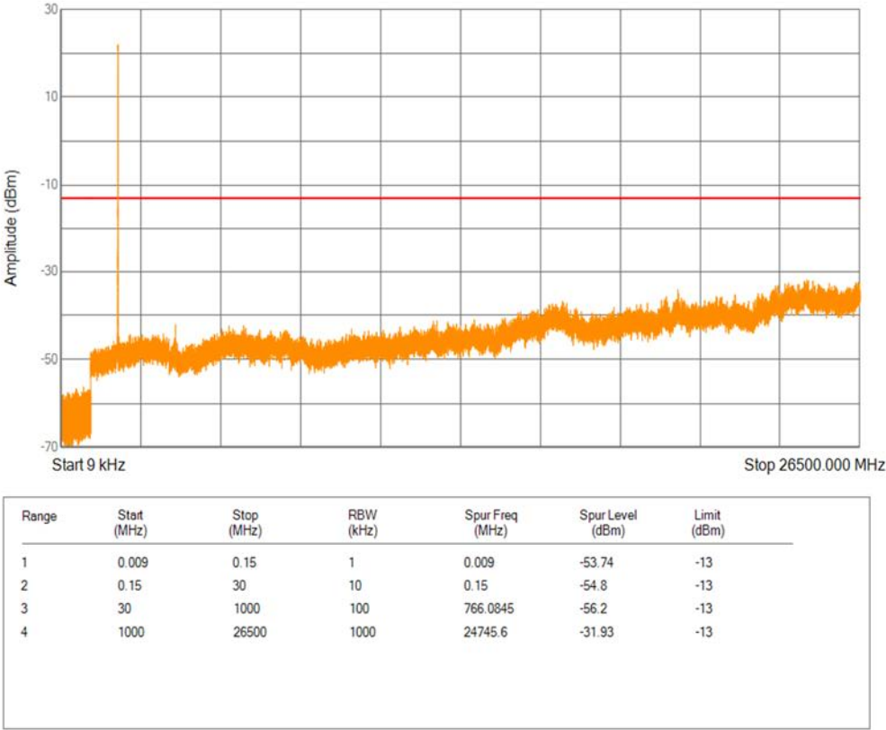
Band2 QPSK BW=10MHz Channel=18650 RB Size=1 Position=#0
