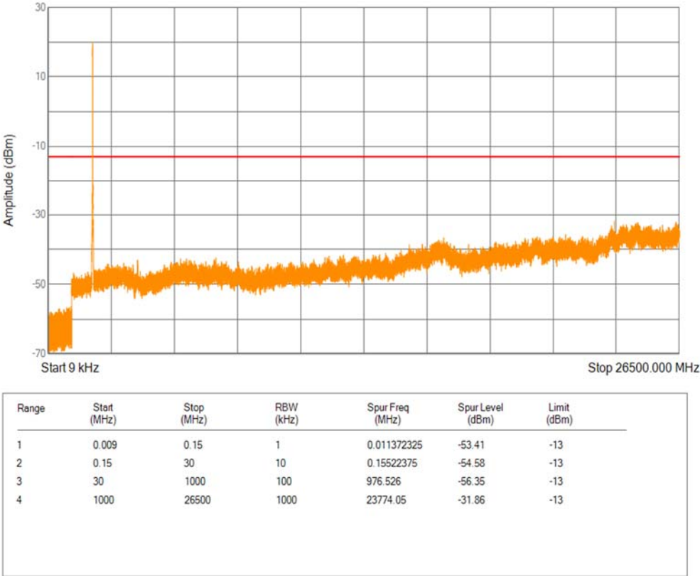
Band2 QPSK BW=15MHz Channel=19125 RB Size=1 Position=#0
