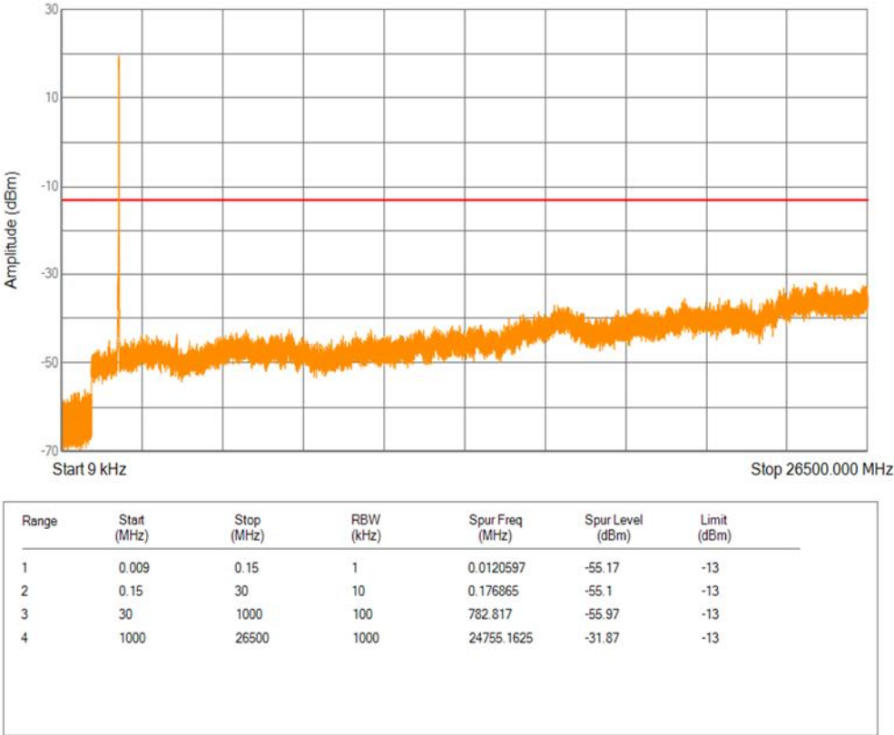
Band2 QPSK BW=20MHz Channel=18700 RB Size=1 Position=#0
