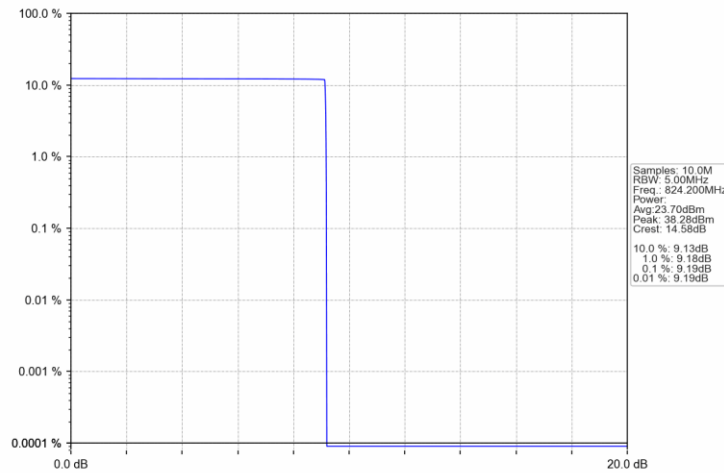
GSM850 GSM LCH 824.2MHz GSM_NTNV
