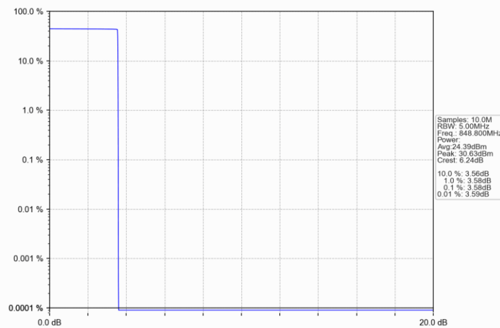
GSM850_GPRS_HCH_848.8MHz_4 TX Slots_NTNV
