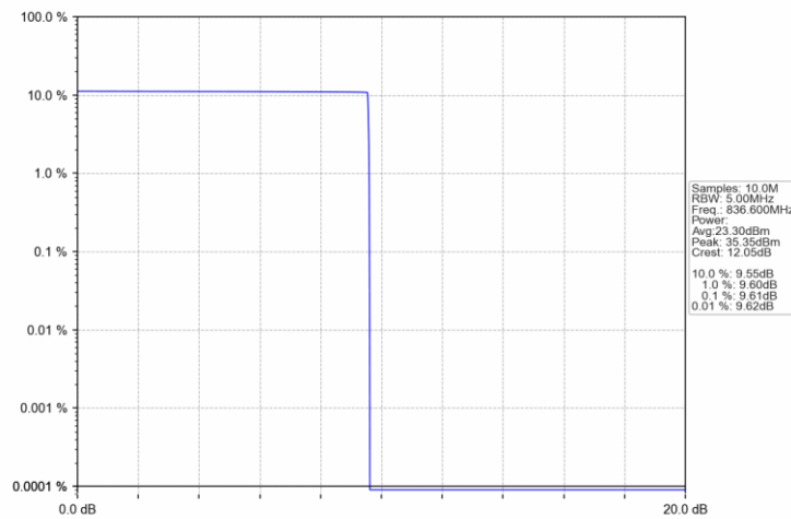
GSM850 GSM MCH 836.6MHz GSM_NTNV
