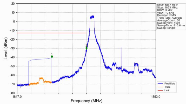
Band2_3MHz_QPSK_LCH_1851.5MHz_RB_1_0_NTNV
