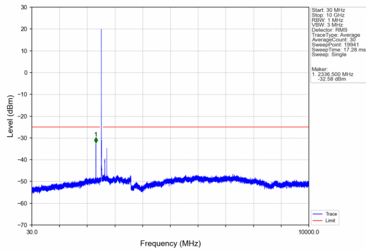
Band7_10MHz_QPSK_MCH_2535MHz_RB_1_0_NTNV
