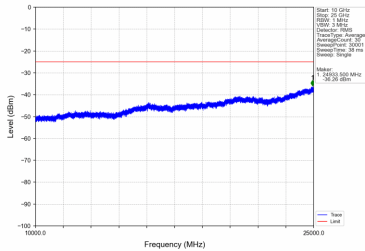
Band7_5MHz_QPSK_LCH_2502.5MHz_RB_1_0_NTNV
