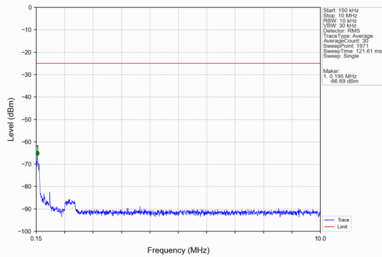
Band7_10MHz_QPSK_HCH_2565MHz_RB_1_0_NTNV
