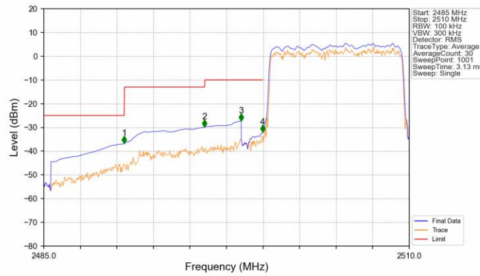
Band7_10MHz_QPSK_LCH_2505MHz_RB_50_0_NTNV
