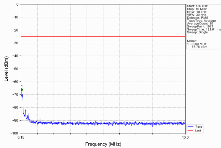
Band7_10MHz_QPSK_MCH_2535MHz_RB_1_0_NTNV
