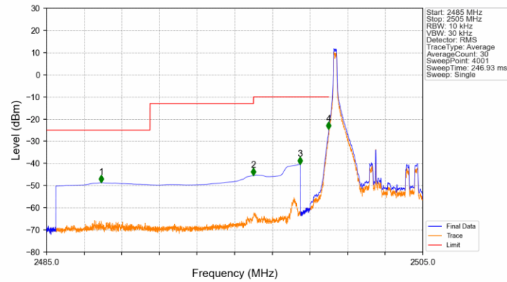
Band7_5MHz_QPSK_LCH_2502.5MHz_RB_1_0_NTNV
