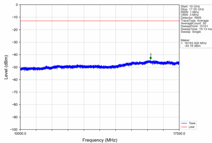
Band4_HSUPA_LCH_1712.4MHz_Subtest 1_NTNV
