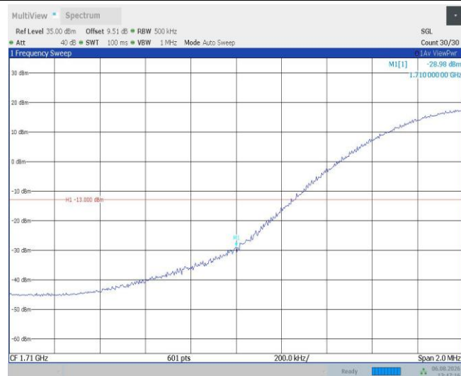
Band66-20MHz-16QAM-132072-1RB#99
