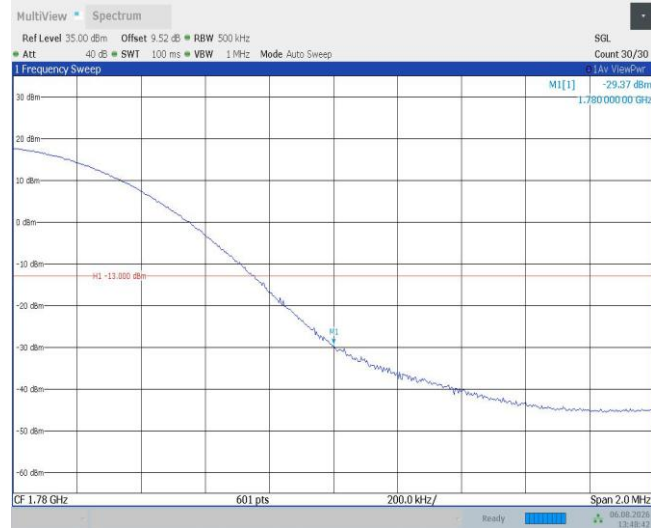
Band66-20MHz-QPSK-132572-100RB#0
