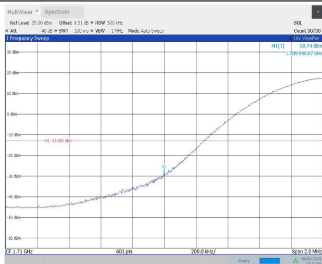
Band66-20MHz-QPSK-132072-1RB#99
