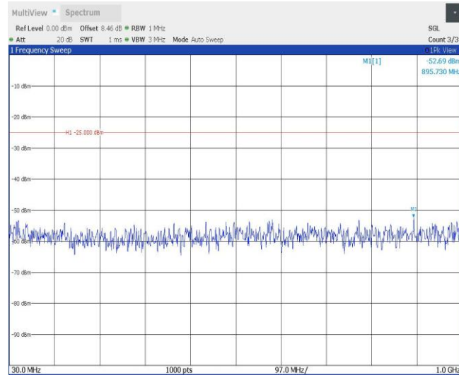
Band41-20MHz-QPSK-40690-1RB#0-Range2:1000~3000MHz
