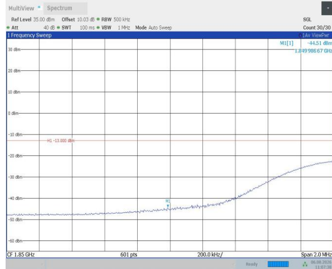
Band2-20MHz-QPSK-18700-100RB#0
