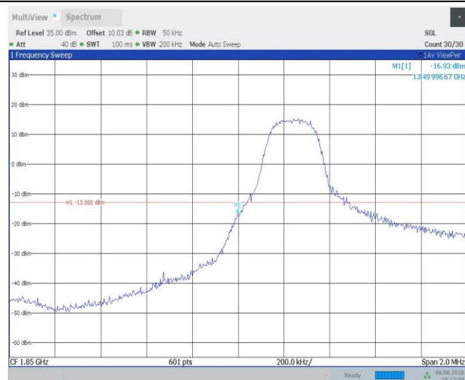
Band2-3MHz-QPSK-18615-1RB#14
