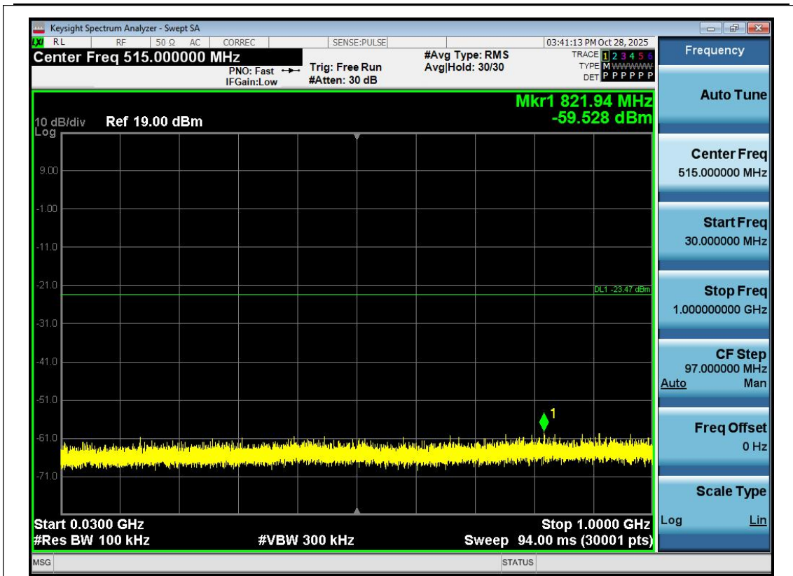
BLE_2M-Ant1-2402-30~1000-PASS
