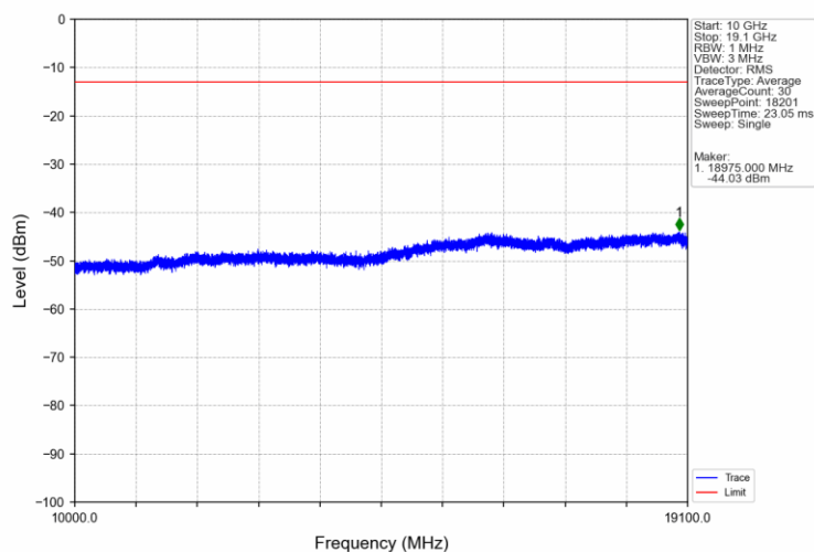
Band2 10MHz QPSK HCH 1905MHz RB 1 49 NTNV
