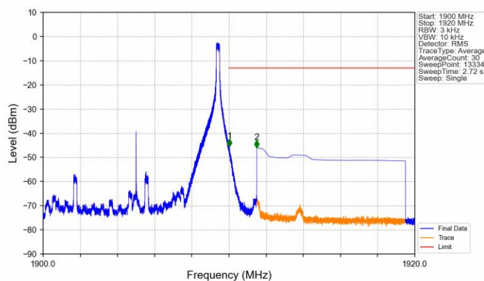
Band2 10MHz QPSK HCH 1905MHz RB 1 49 NTNV
