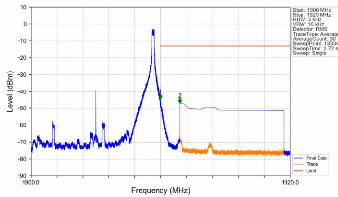
Band2 10MHz 16QAM HCH 1905MHz RB 1 49 NTNV
