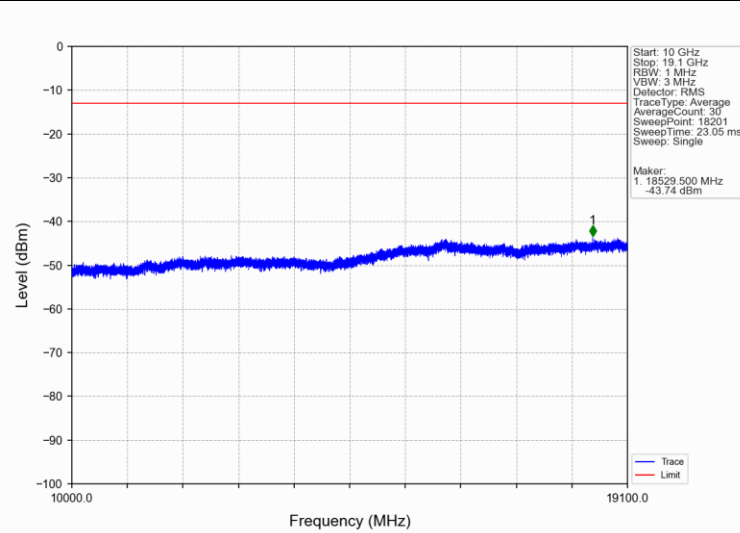
Band2 10MHz 16QAM HCH 1905MHz RB 1 0 NTNV
