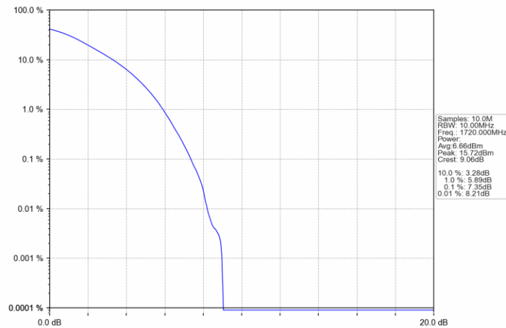
Band66 20MHz 16QAM LCH 1720MHz RB 27 0 NTNV
