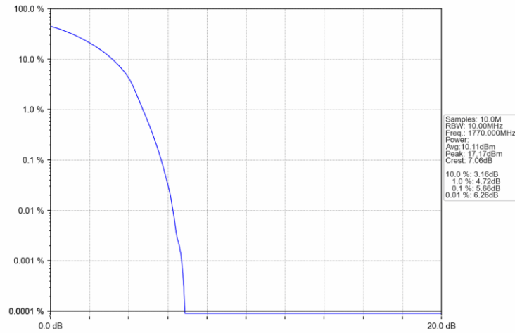
Band66 20MHz QPSK HCH 1770MHz RB 100 0 NTNV
