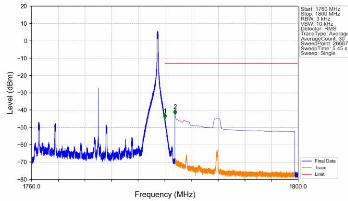
Band66 20MHz 16QAM HCH 1770MHz RB 1 99 NTNV
