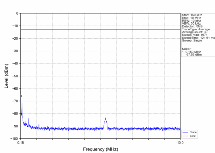
Band66_20MHz_16QAM_LCH_1720MHz_RB_1_0_NTNV
