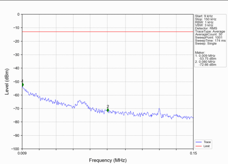
Band66_20MHz_16QAM_LCH_1720MHz_RB_1_0_NTNV
