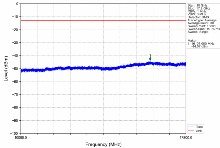
Band66 20MHz 16QAM HCH 1770MHz RB 1 99 NTNV
