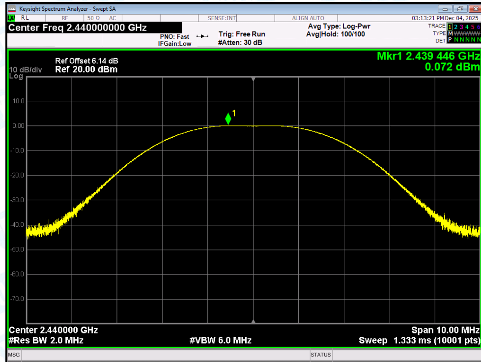
Power NVNT BLE 2Mbps 2440MHz Ant1
