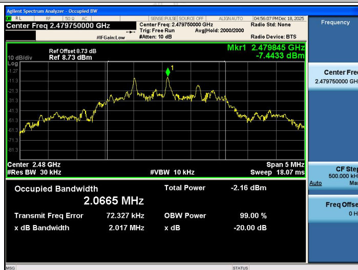
GFSK_Ant1_2479.75
