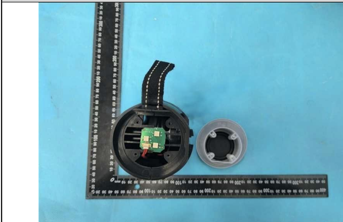
EUT Photo
