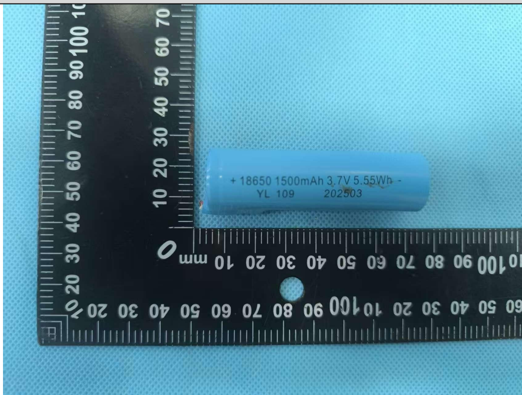
EUT Photo
