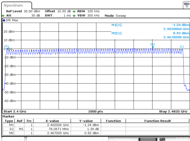
2EDR_DH1_Hopping
