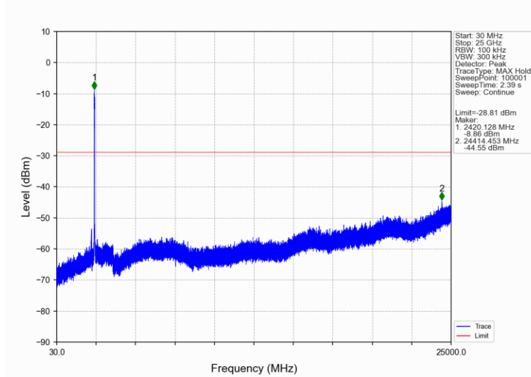
802.11n(HT40)_LCH_2422MHz_Ant1 (SISO)_NTNV
