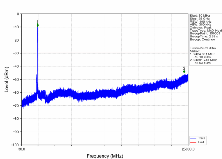
802.11n(HT40)_MCH_2437MHz_Ant1 (SISO)_NTNV
