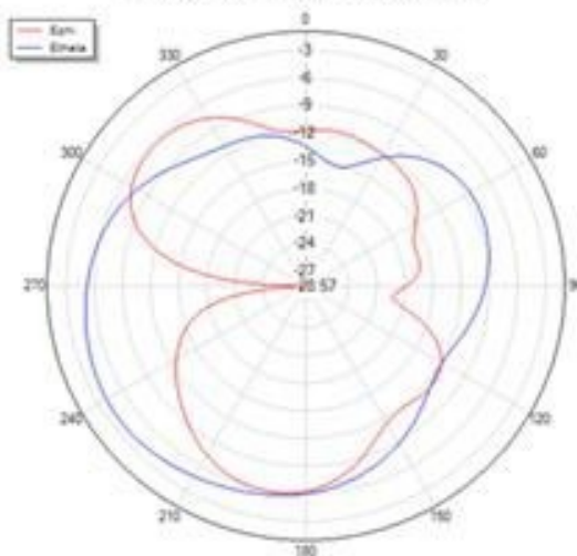
Theta=90 freq=2500MHz
