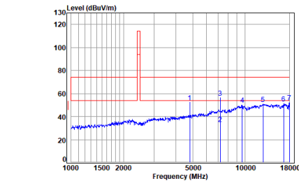
2.4G_SRD_LOW_TX_Horizontal
