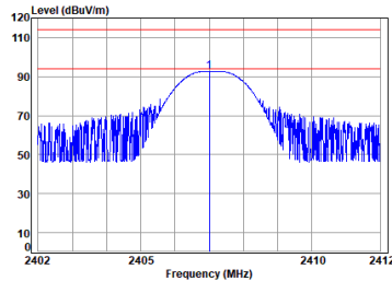
2.4G_SRD_LOW_TX_Horizontal
