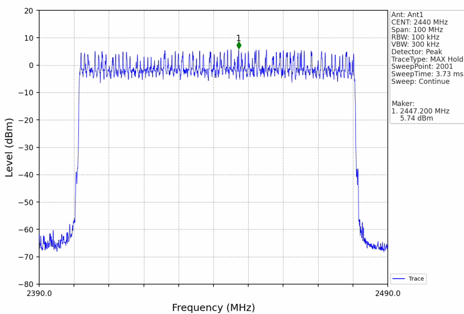
8DPSK_3DH5_HOPP_Ant1_NTNV
