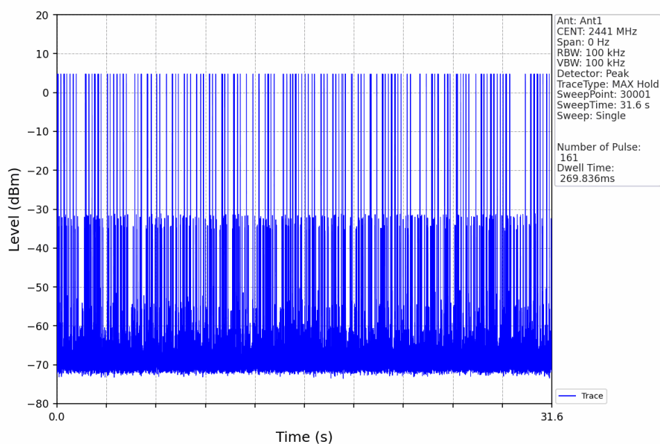
Pi/4DQPSK_2DH3_HOPP_Ant1_NTNV
