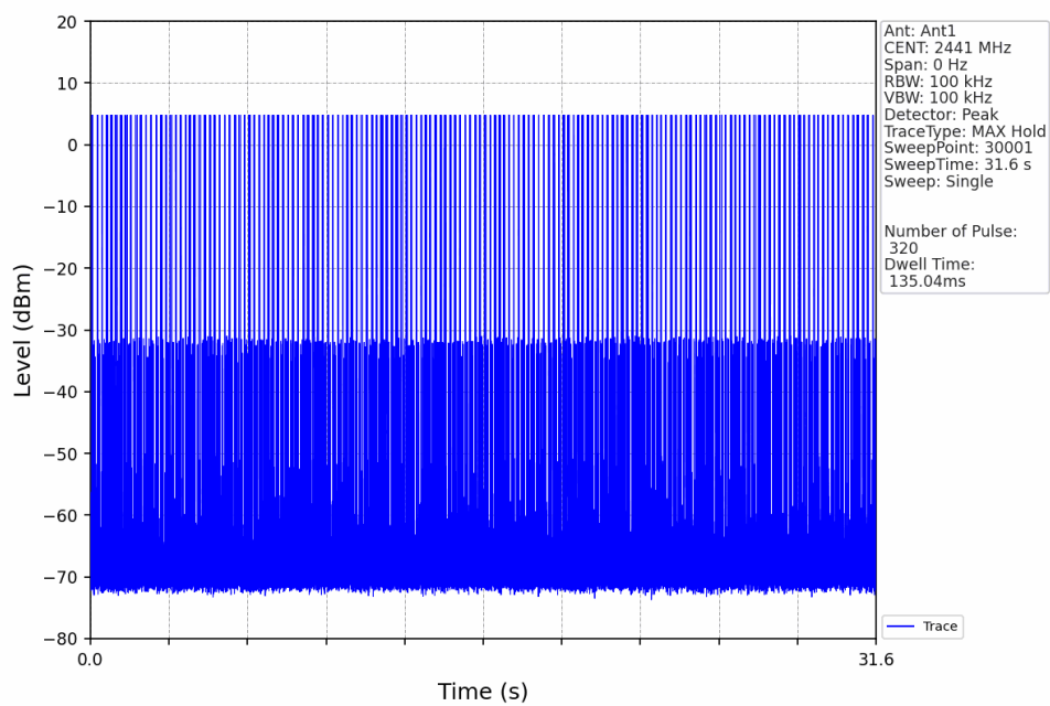
Pi/4DQPSK 2DH1_HOPP_Ant1_NTNV
