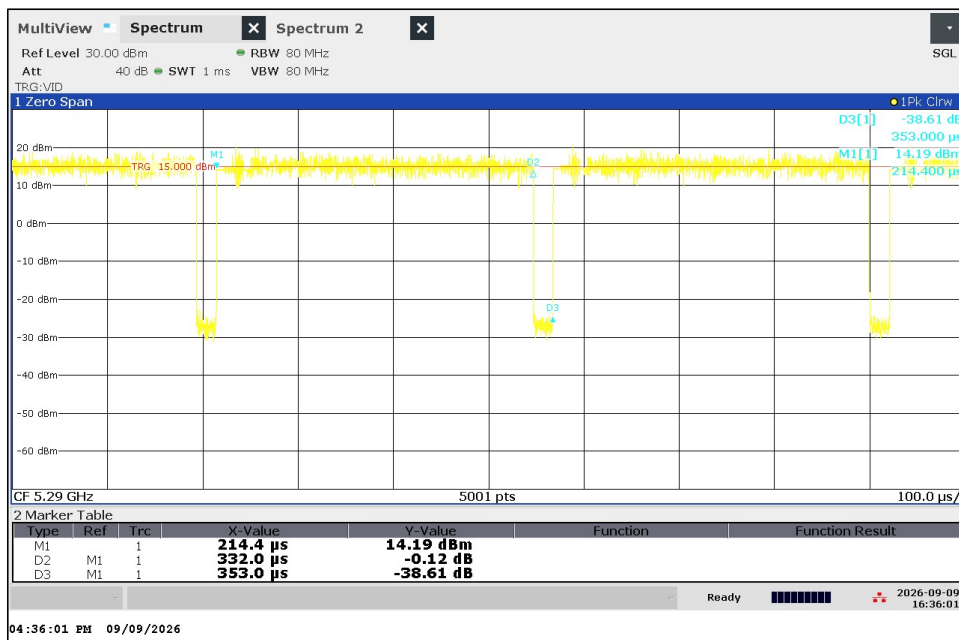
802.11ac VHT0 5290 MHz Duty Cycle
