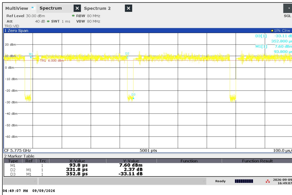
802.11ac VHT0 5775 MHz Duty Cycle
