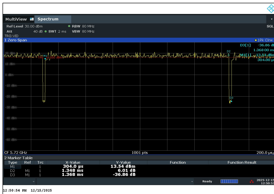
802.11ac VHT0 5720 MHz Duty Cycle
