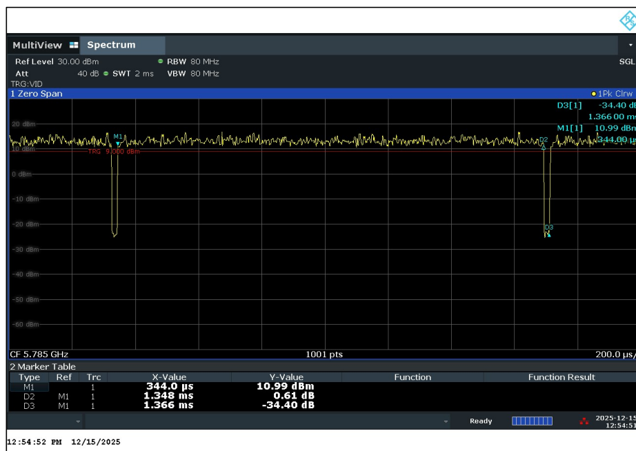
802.11ac VHT0 5785 MHz Duty Cycle
