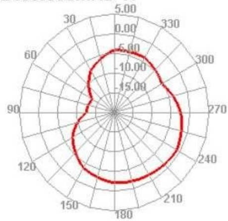
2450.000MHz H
