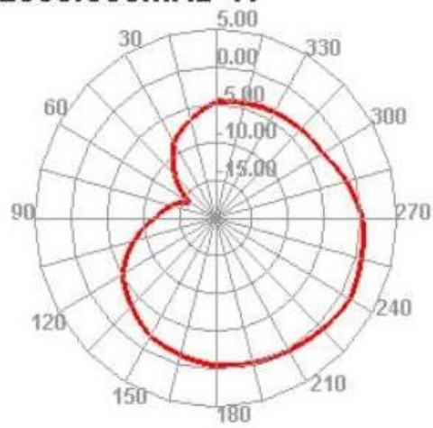
2500.000MHz H
