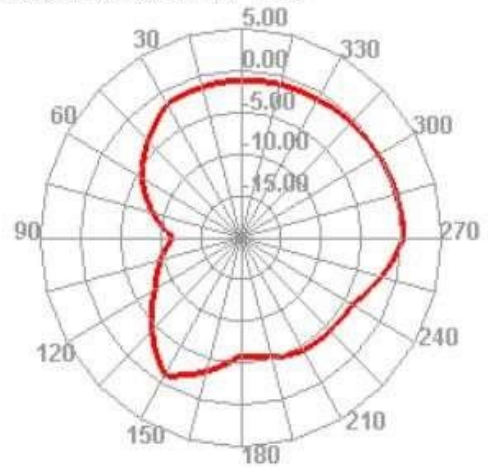
2500.000MHz E2
