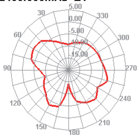
2450.000MHz E1
