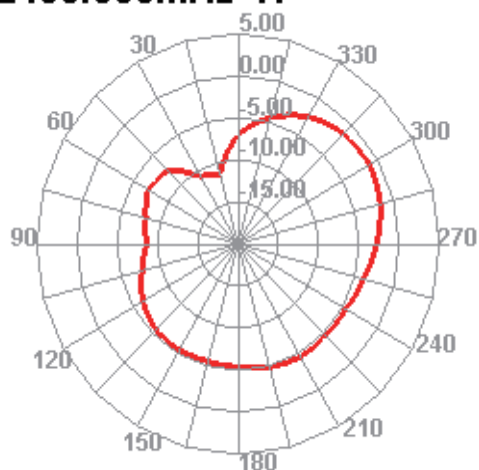
2400.000MHz H
