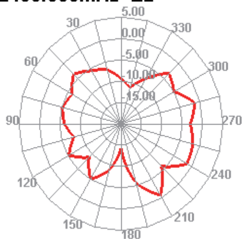
2450.000MHz E2
