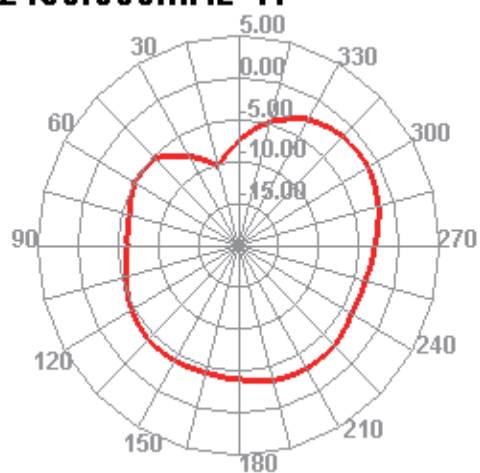
2450.000MHz H
