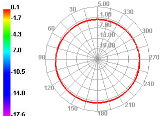
2400.000MHz H
