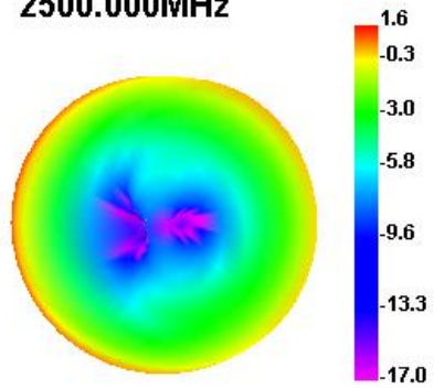
2500.000MHz
