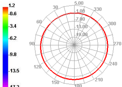
2450.000MHz H
