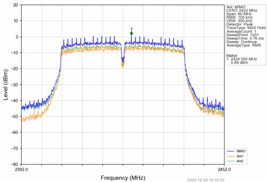
802.11n(HT40)_LCH_2422MHz_MIMO_NTNV
