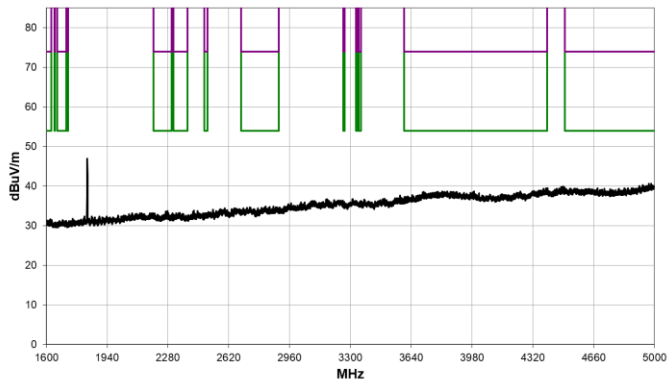
1.6 GHz – 5 GHz
