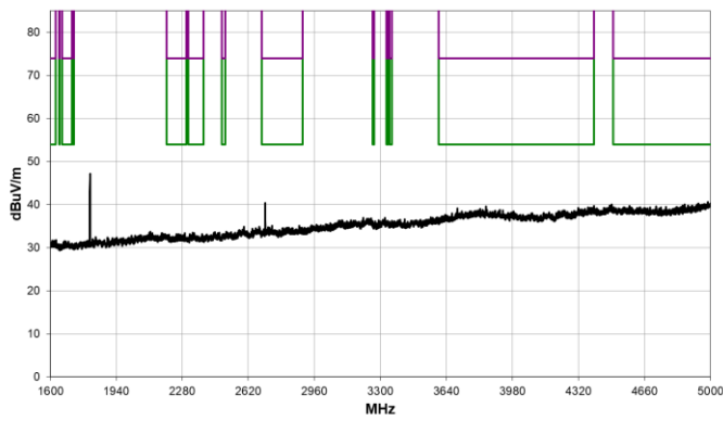
1.6 GHz – 5 GHz
