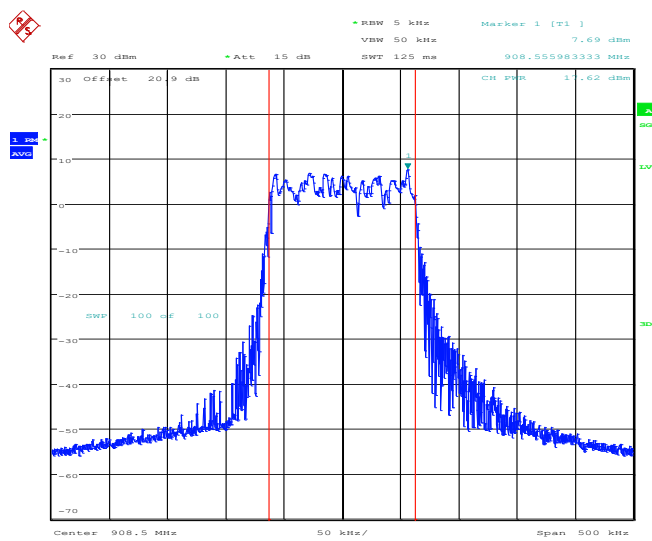
908.5 MHz
