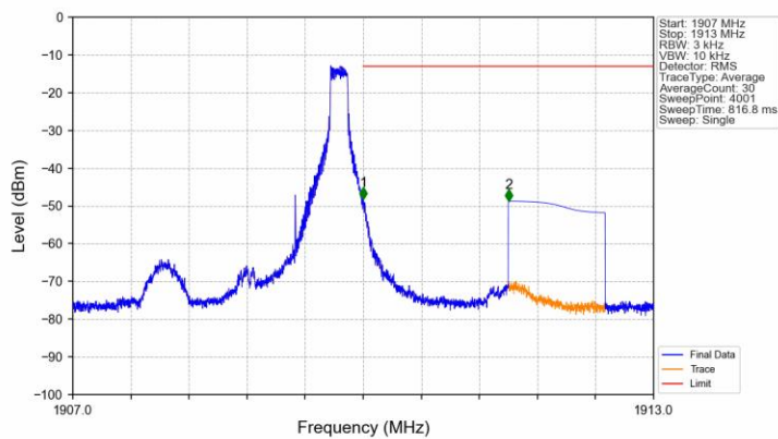
Band2_1.4MHz_QPSK_HCH_1909.3MHz_RB_1_5_NTNV
