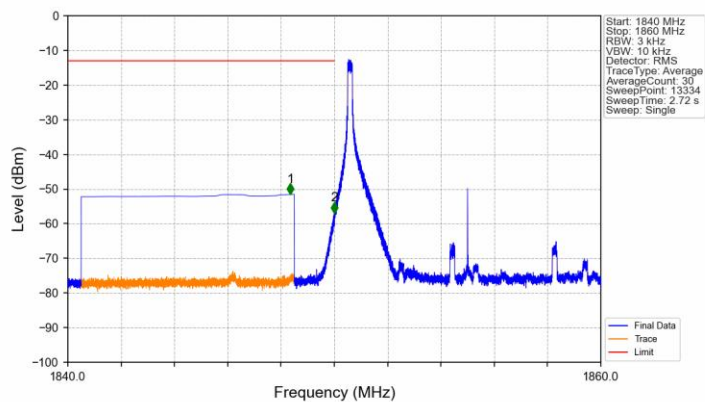
Band2_10MHz_QPSK_LCH_1855MHz_RB_1_0_NTNV
