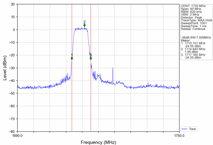
Band4_20MHz_16QAM_LCH_1720MHz_RB_27_0_NTNV
