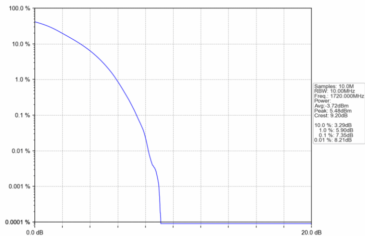
Band4_20MHz_16QAM_LCH_1720MHz_RB_27_0_NTNV
