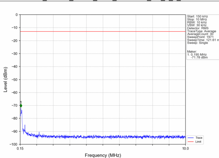
Band4_10MHz_QPSK_HCH_1750MHz_RB_1_0_NTNV
