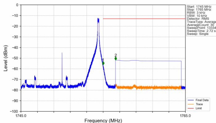
Band4_10MHz_QPSK_HCH_1750MHz_RB_1_49_NTNV
