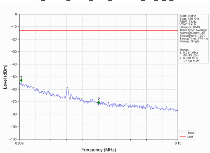
Band4_10MHz_QPSK_HCH_1750MHz_RB_1_0_NTNV
