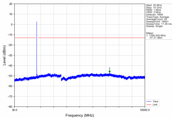
Band4_20MHz_QPSK_MCH_1732.5MHz_RB_1_0_NTNV
