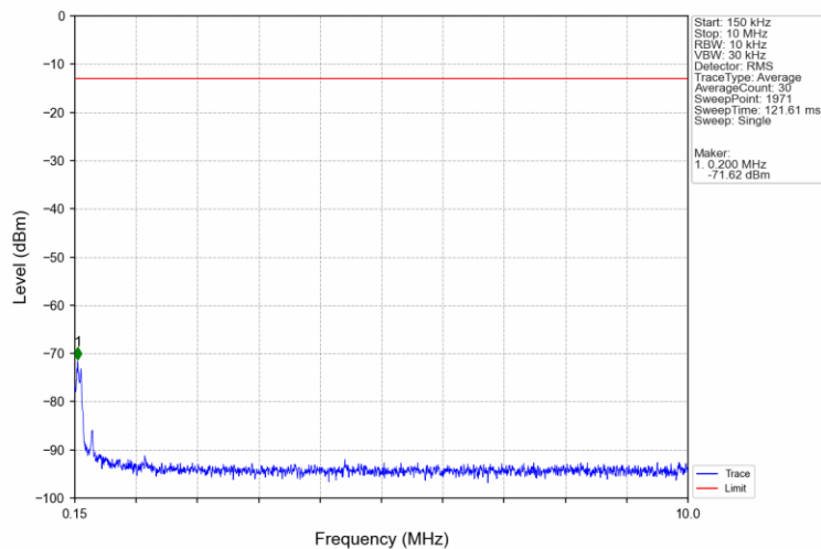
Band4_20MHz_16QAM_LCH_1720MHz_RB_1_0_NTNV
