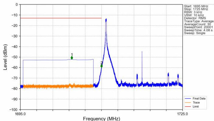
Band4 15MHz QPSK LCH 1717.5MHz RB 1 0 NTNV
