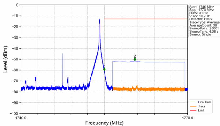
Band4_15MHz_QPSK_HCH_1747.5MHz_RB_1_74_NTNV
