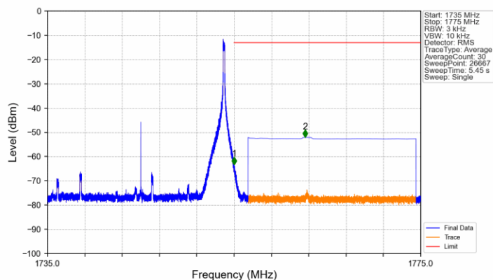
Band4_20MHz_QPSK_HCH_1745MHz_RB_1_99_NTNV
