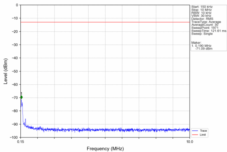
Band4_20MHz_QPSK_MCH_1732.5MHz_RB_1_0_NTNV
