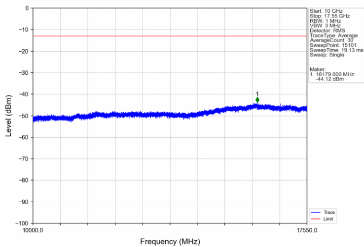
Band4_15MHz_QPSK_HCH_1747.5MHz_RB_1_74_NTNV
