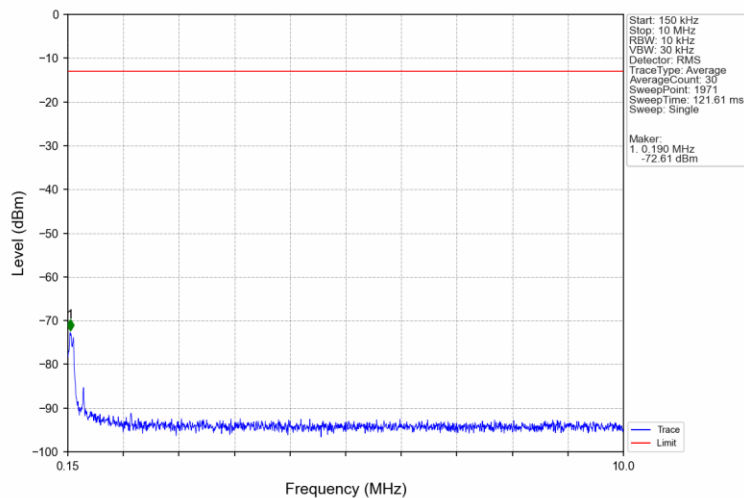
Band4_20MHz_QPSK_HCH_1745MHz_RB_1_0_NTNV
