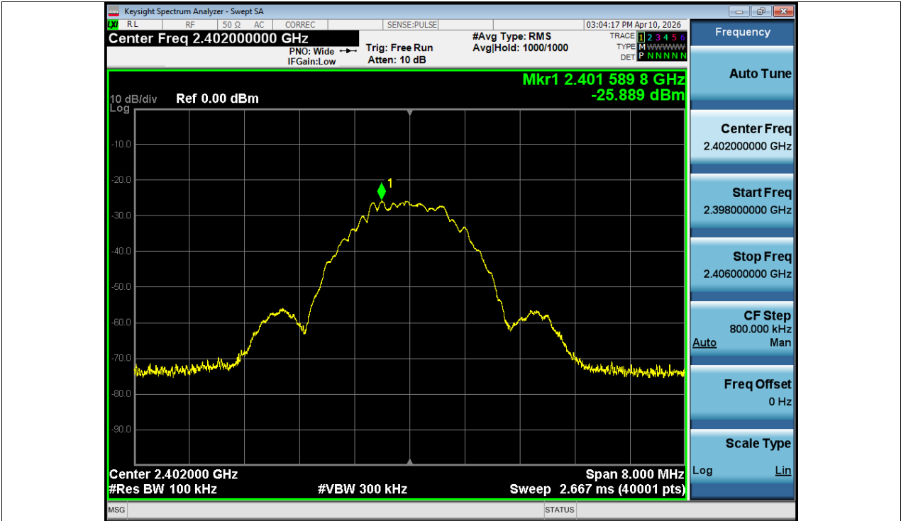
Tx. Spurious NVNT BLE 2M 2402MHz Ant1 Ref
