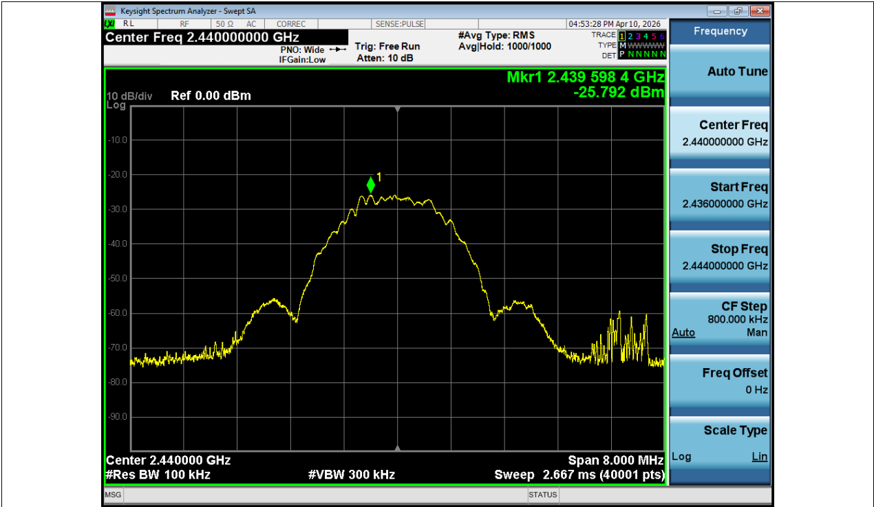
Tx. Spurious NVNT BLE 2M 2440MHz Ant1 Ref
