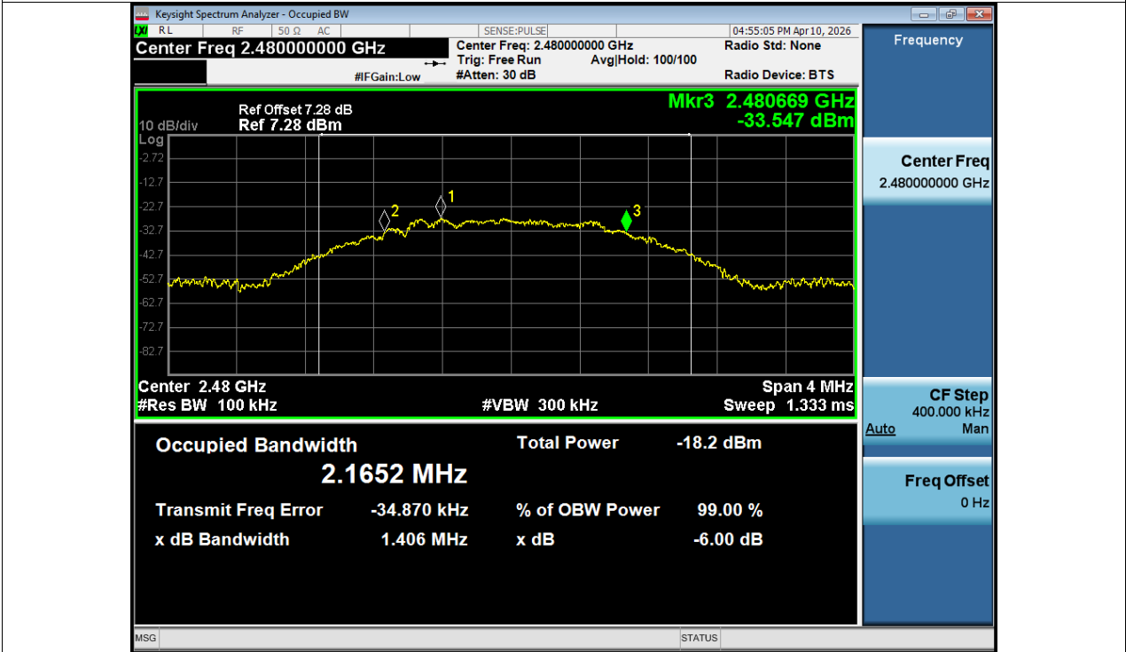
-6dB Bandwidth NVNT BLE 2M 2480MHz Ant1
