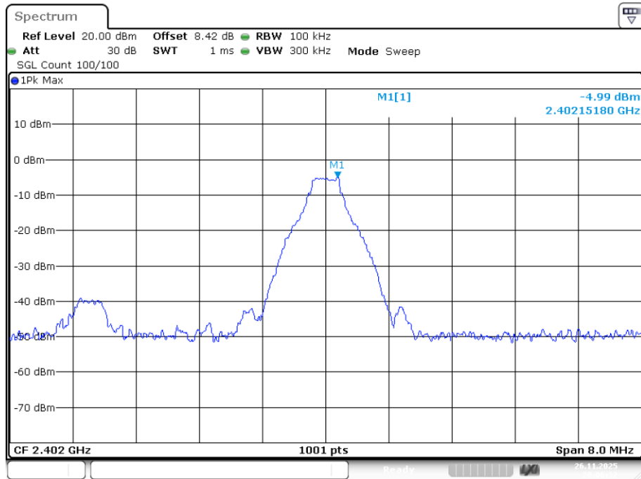
Band Edge NVNT GFSK 2402MHz Ant1 No-Hopping Ref
