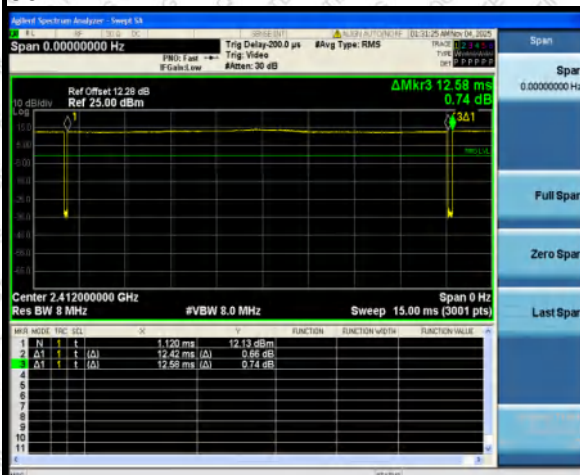
802.11n HT20
