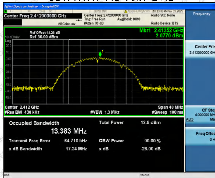
OBW NVNT 11B Ant1 2412
