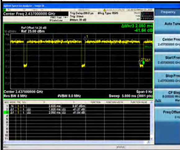
802.11n HT20
