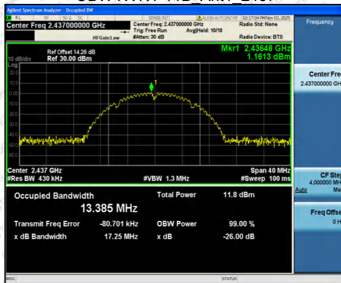
OBW NVNT 11B Ant1 2437
