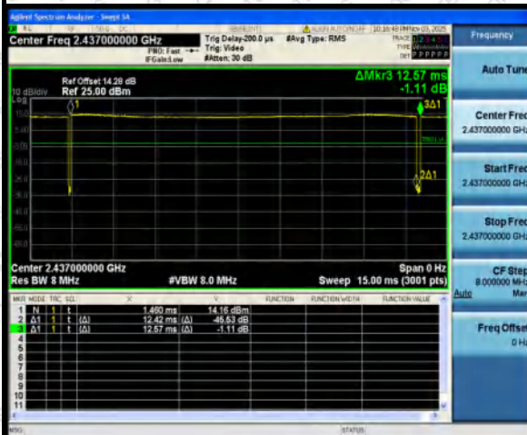
802.11n HT20
