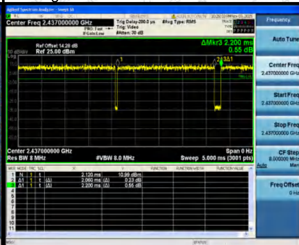
802.11n HT40
