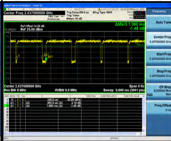
802.11n HT40
