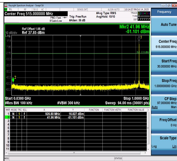
TURMASS-Ant1-926.8-30~1000-PASS
