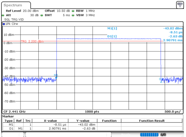
DH5_Hopping
