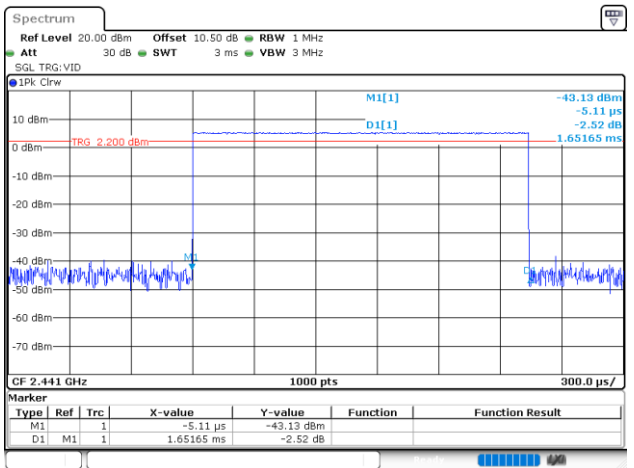
DH3_Hopping
