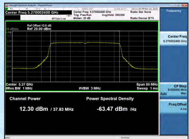
11AX40MIMO-Ant8-5270-PASS
