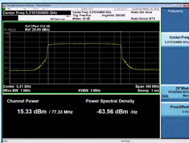
11AX80SISO-Ant6-5210-PASS
