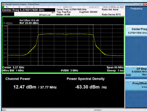
11AX40MIMO-Ant6-5270-PASS
