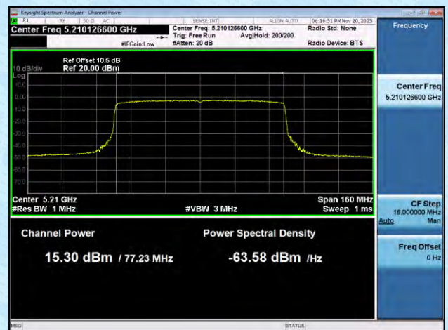
11AX80SISO-Ant8-5210-PASS
