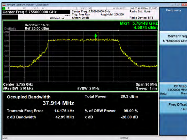
11AX40MIMO-Ant6-5755
