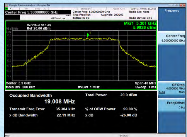
11AX20MIMO-Ant8-5300
