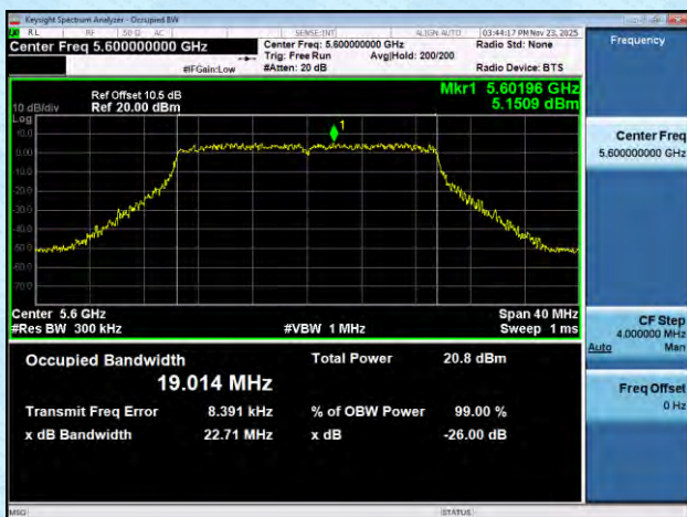
11AX20MIMO-Ant6-5600
