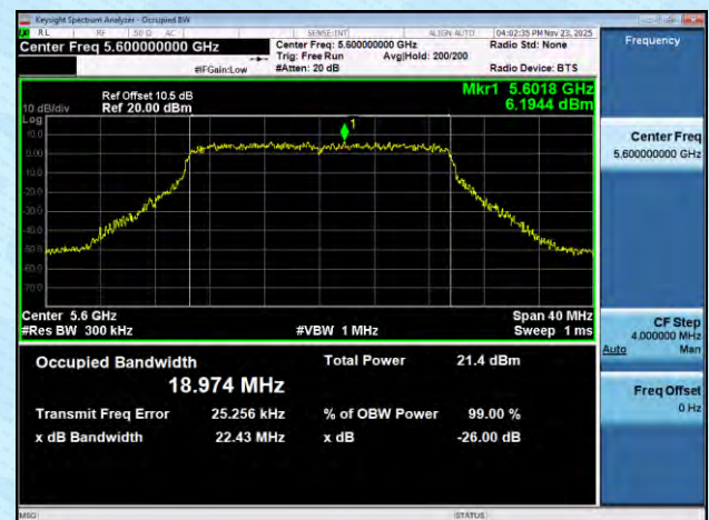
11AX20MIMO-Ant8-5600
