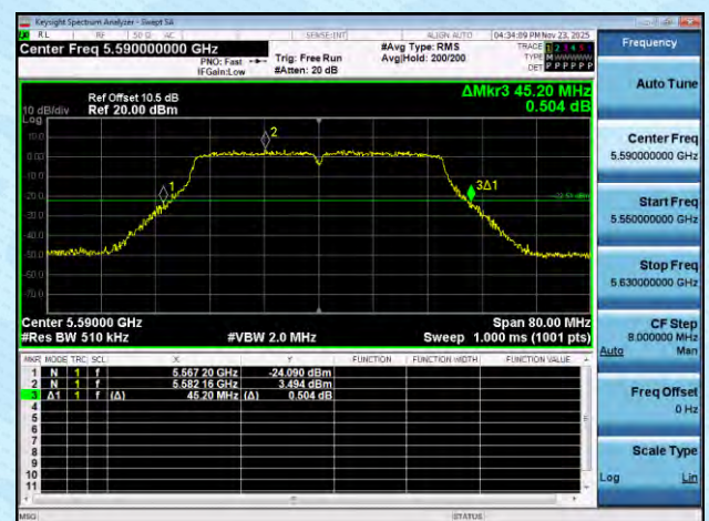
11N40MIMO-Ant8-5590
