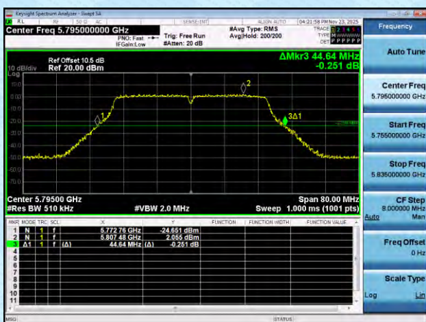
11N40MIMO-Ant6-5795
