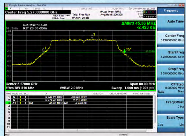
11N40MIMO-Ant8-5270
