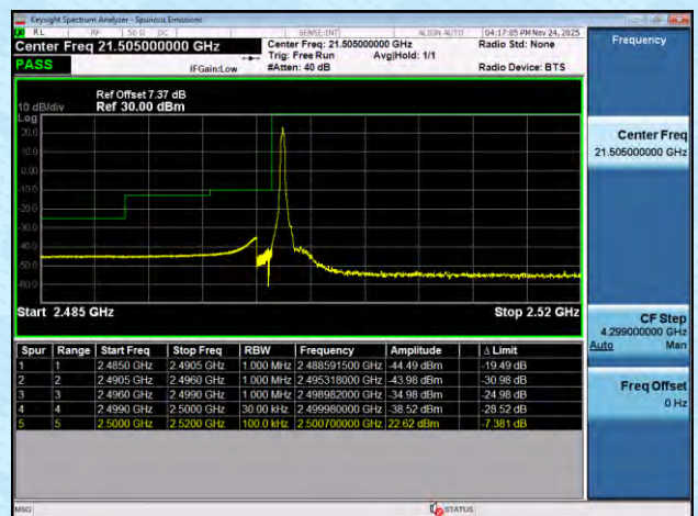
NTNV-n7-PC3-15-30-L-DFT-BPSK-Edge_1RB_Left-PASS
