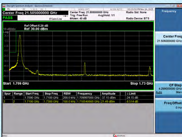
NTNV-n66-PC3-15-20-L-DFT-BPSK-Edge_1RB_Left-PASS
