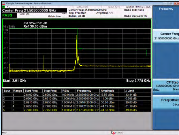
NTNV-n41-PC2-30-90-L-DFT-BPSK-Edge_1RB_Left-PASS
