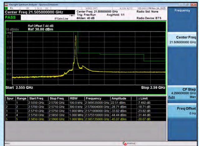
NTNV-n7-PC3-15-20-L-DFT-BPSK-Edge_1RB_Left-PASS
