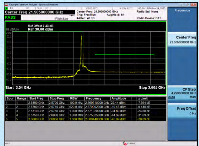
NTNV-n7-PC3-15-40-L-DFT-BPSK-Edge_1RB_Left-PASS
