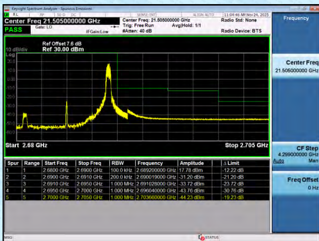
NTNV-n41-PC2-30-20-L-DFT-BPSK-Edge_1RB_Left-PASS
