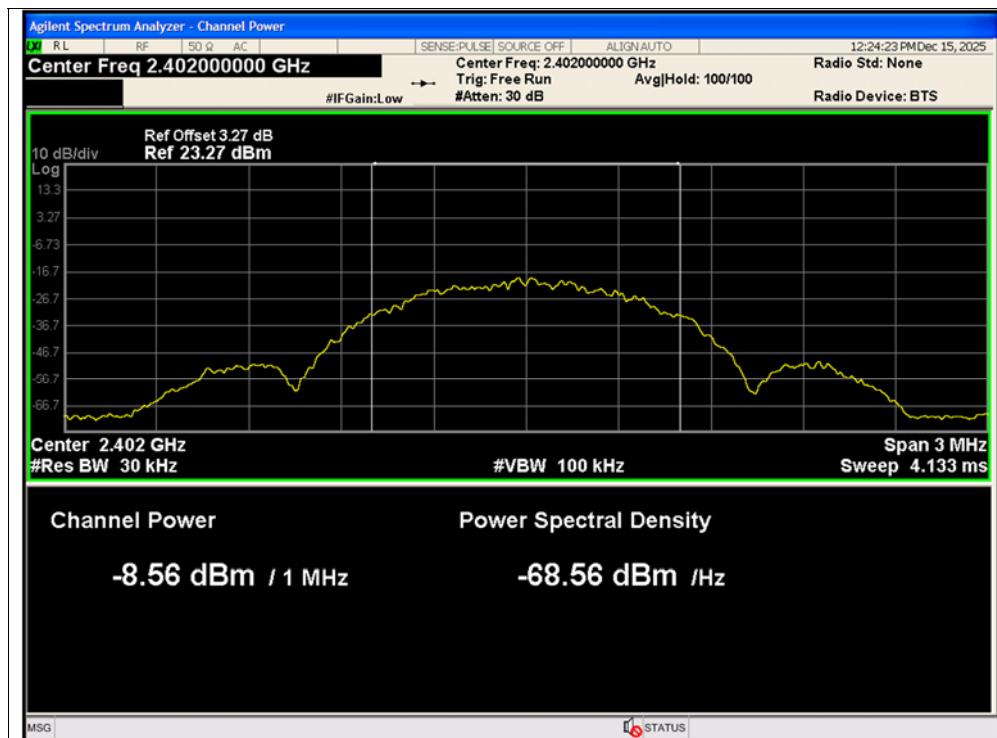
Average Power NVNT BLE 1M 2402MHz Ant1
