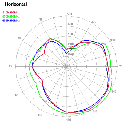
5150~5850MHz
