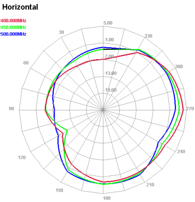
2400~2500MHz
